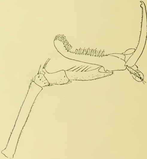
Fig. 1. Neodryinus sumatranus nov. spec. ♀. Rechter Vorderfuß. 55 : 1.
