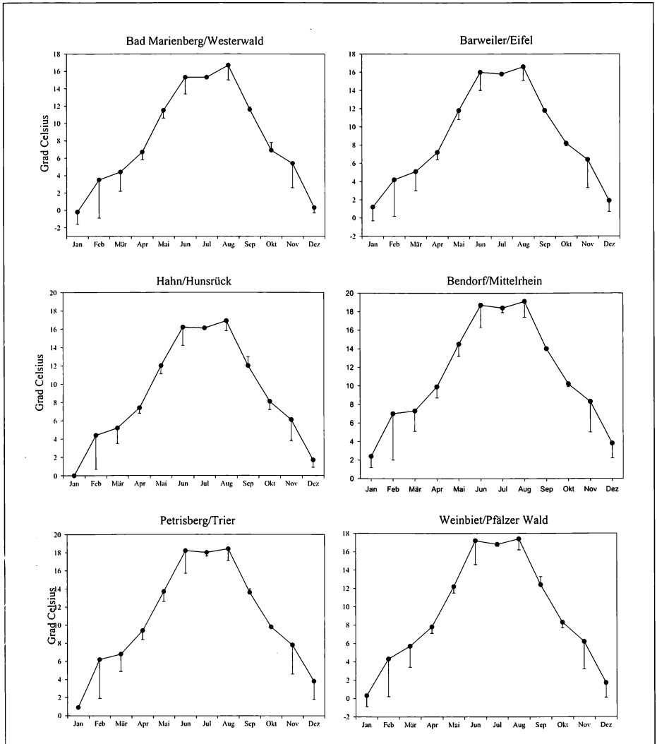
Abb. 7: Monatsmittelwerte der Temperatur an sechs verschiedenen Stationen in Rheinland-Pfalz 2002. Die Fehlerbalken geben die Abweichung vom langjährigen Mittel der letzten 30 Jahre an. [Quelle: DWD.]
