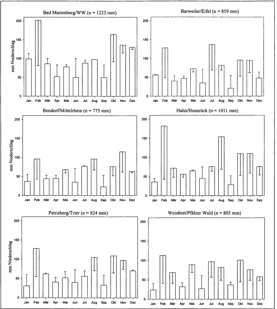
Abb. 8: Monatliche Niederschlagssummen an sechs verschiedenen Stationen in Rheinland-Pfalz 2002. Die Fehlerbalken geben die Abweichung vom langjährigen Mittel der letzten 30 Jahre an. [Quelle: DWD.]
