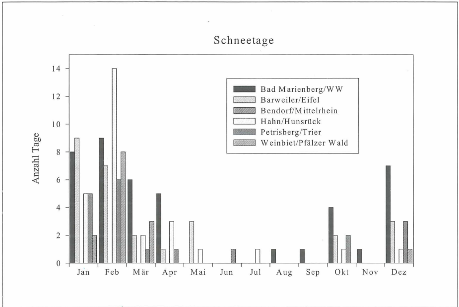
Abb. 9: Anzahl der Tage mit festen Niederschlägen (Schnee, Hagel und Graupel) pro Monat an sechs verschiedenen Stationen in Rheinland-Pfalz 2002. [Quelle: DWD.]
