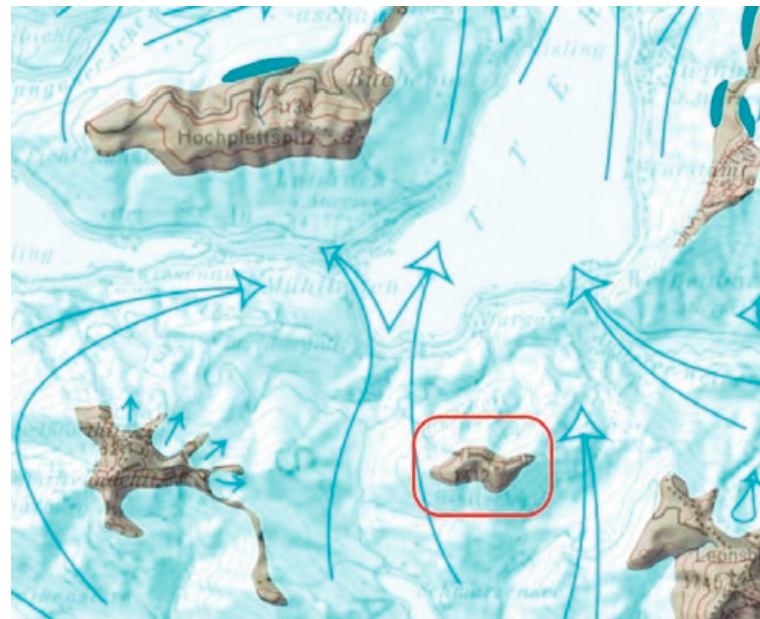
ABB. 14: Eisströme am S-Ende des Attersees mit dem Untersuchungsgebiet (roter Rahmen, dessen Breite 2,5 km entspricht) während des letzteiszeitlichen Maximums nach VAN HUSEN & EGGER (2014)
