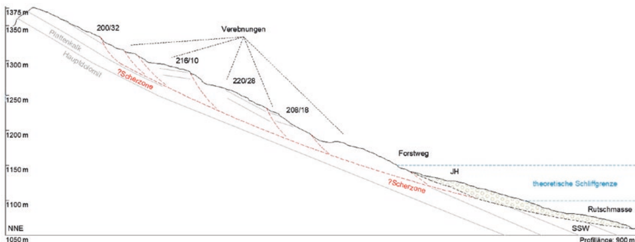
ABB. 11: Schematisches Profil durch die Breitenbergalm-Massenbewegung (3) mit der vermuteten Scherzone, Fallrichtung/Fallwinkel der Schichtflächen und der Schließgrenze des letzteiszeitlichen Maximums (nach VAN HUSEN, 1987). Die Lage des Profils ist in Abb. 1 ersichtlich. FIG. 11: Schematic cross section of the Breitenbergalm slope deformation (3) with the assumed shear zone, dip direction/dip angle of bedding planes and trimline of the last glacial maximum (according to VAN HUSEN, 1987). The position of the cross section is shown in fig. 1.
