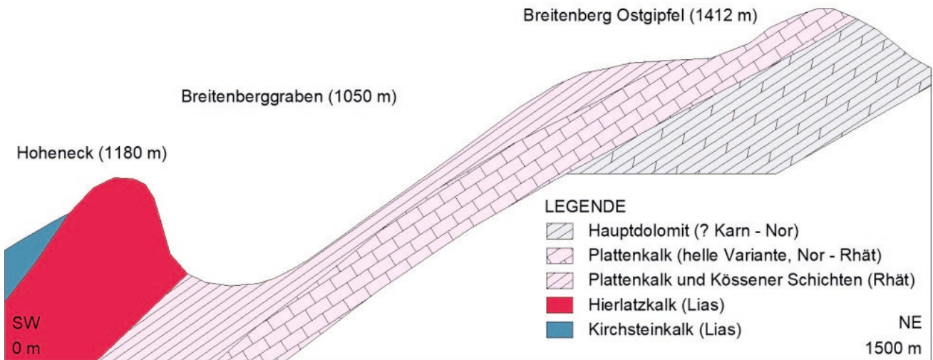
ABB. 3: Geologisches Profil aus SPENGLER (1911). Die Benennung der Liaskalke erfolgt nach VAN HUSEN (1989). Die Lage des Profils ist in Abb. 1 ersichtlich. FIG. 3: Geological cross section according to SPENGLER (1911). The naming of the Lias limestones follows VAN HUSEN (1989). The position of the cross section is shown in fig. 1.
