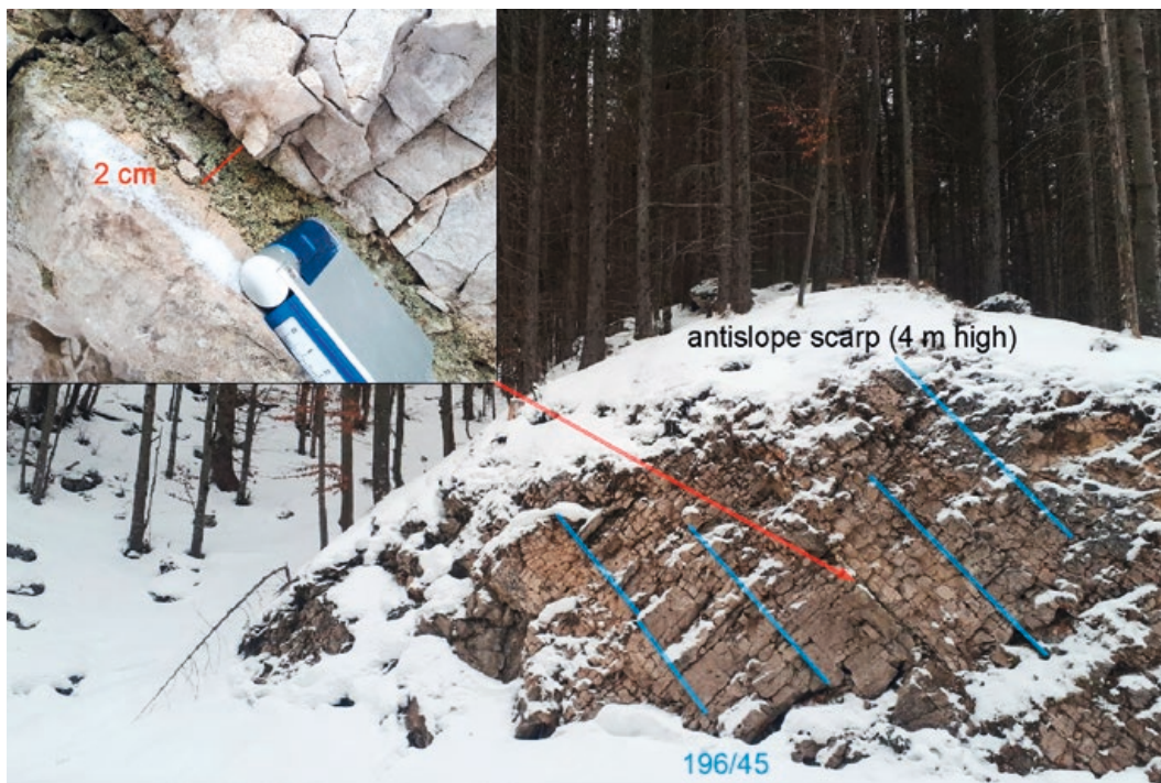
ABB. 15: Verwitterte Mergelzwischenlage im SSW-fallenden Plattenkalk, die in einem Anschnitt der Forststraße am SSW-Hang (Nackental, 915 m SH) freigelegt wurde.
