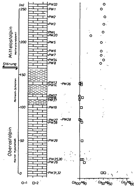
Abb. 5: Ca/Mg-Verhältnis der Karbonate im Profil an der Pfriemeswand 1 = Mittelostalpin 2 = Oberostalpin
