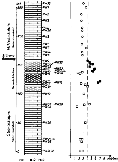
Abb. 2: Werte für die Halbhöhenbreite des 10-Å-Illit-Reflexes in Abhängigkeit zur Lage im Profil an der Pfirmeswand (gestrichelte Gerade = Regressionsgerade). 1 = mittelostalpine Karbonatgesteine 2 = oberostalpine Mergel 3 = oberostalpine Karbonatgesteine
