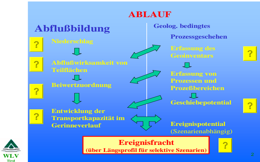
Abb. 6: Übersicht des Ablaufes zur Anschätzung der Ereignisfracht in Wildbacheinzugsgebieten
