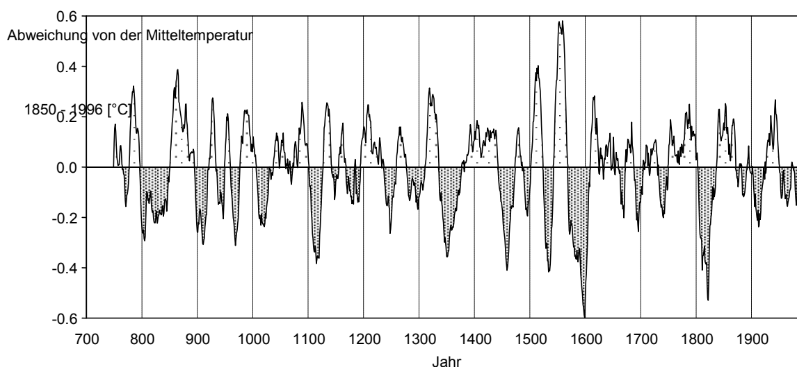
Abb. 9: Rekonstruktion der Abweichung der Sommertemperatur (Juni-Juli) der letzten 1250 Jahre vom Mittel der Jahre 1850-1996 (geglättet mit einem gleitenden Mittel über 20 Perioden).
