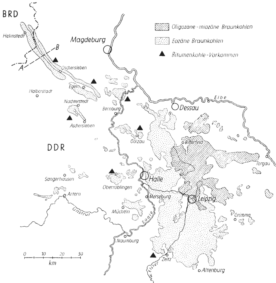
Abb. 1. Die paläogenen Braunkohlenvorkommen westlich der Elbe und ihre Bitumenkohlevorkommen
