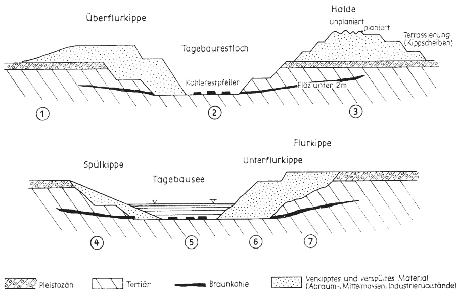
Abb. 2. Die morphologischen Strukturformen des Braunkohlenbergbaues in den Tagebaugebieten westlich der Elbe am Beispiel „Braunkohlevorkommen Geiseltal“ (schematische Darstellung)
