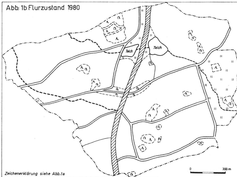
Abb. 1. Charakteristischer Ausschnitt aus dem Moritzburger Kleinkuppengebiet. a) Flurzustand 1960, b) Flurzustand 1980.
