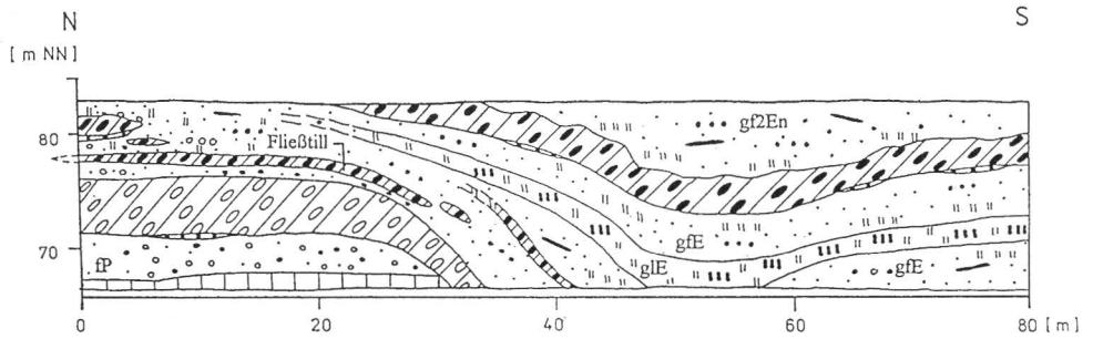
Abb. 4 Randbereich der Burgkennitzer Rinne im Tagebau Gröbern, September 1987, 2. Abraumschnitt (Legende siehe Abb. 9)
