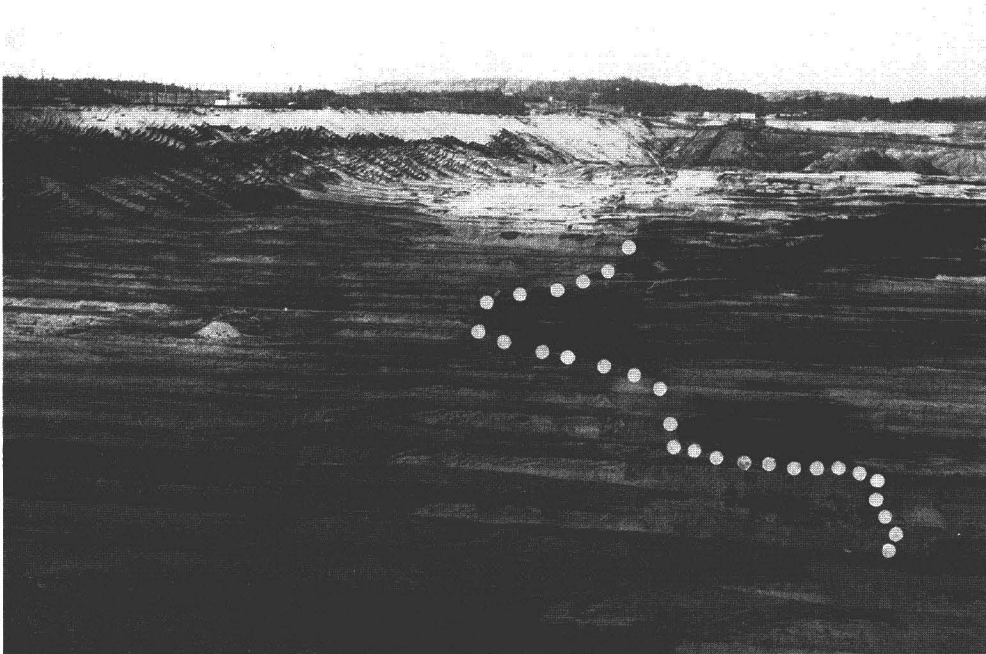
Abb. 2 Nordrand der Burgkennitzer Rinne im Braunkohlentagebau Gröbern, September 1987; links: Schmelzwassersande des Miltitzer Intervalls (Rinnenfüllung), rechts: untermiozäne Braunkohle und Ton
