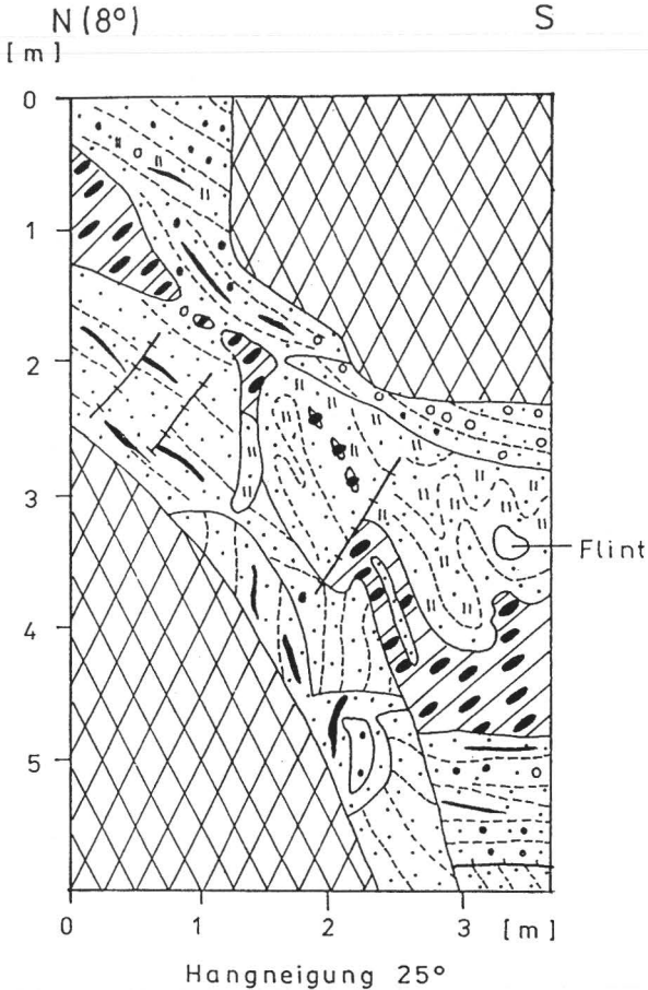
Abb. 8 Elsterzeitlicher Fließstill in Schmelzwassersanden am Rand der Burgkernitzer Rinne im Tagebau Gröbern, September 1987, Böschungswinkel 25^\circ (Legende siehe Abb. 9)
