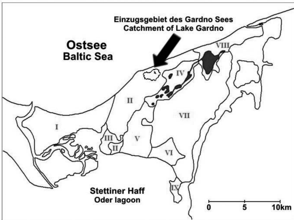
Abb. 1 Einzugsgebiet des Gardno-Sees auf der Insel Wollin vor dem Hintergrund der Physisch-geographischen Regionen (Nordwestpolen): I. Swine-Pforte, II. Wolliner Höhenzug, III. Lebbin–Kalkofen-Hügel, IV. Wolliner Seenplatte, V. Dargebanzer Flachland, VI. Mokratz-Gebirge, VII. Codram-Senkung, VIII. Dievenow-Nehrung, IX. Halbinsel Rów (MARSZ 1967).
