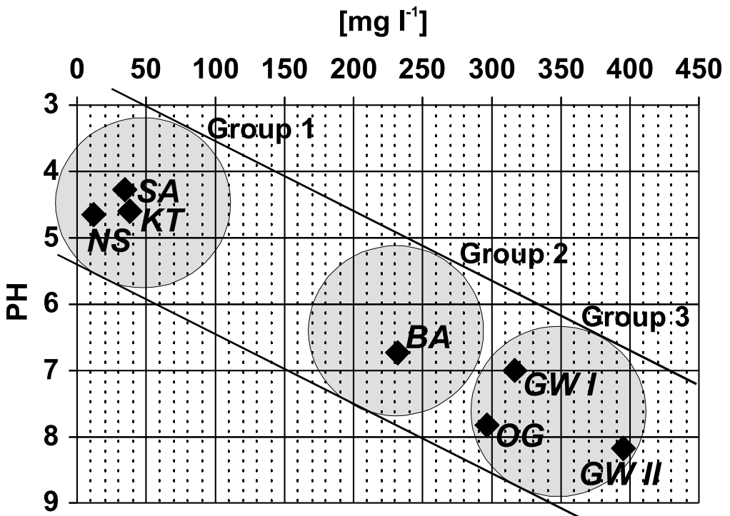
Abb. 8 Hydrochemischen Gruppe des Wasserkreislaufes im Einzugsgebiet des Gardno-Sees. NS = Niederschlag, KT = Kronentraufe, SA = Stammablauf, BA = Bodenabfluss Hänge, OG = Oberirdische Gewässer, GW I = Grundwasser-I-Niveau, GW II = Grundwasser-II-Niveau.
