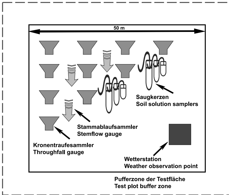
Abb. 3 Waldtestfläche zur Überwachung der Niederschlagstransformation. Einzugsgebiet des Gardno-Sees.
