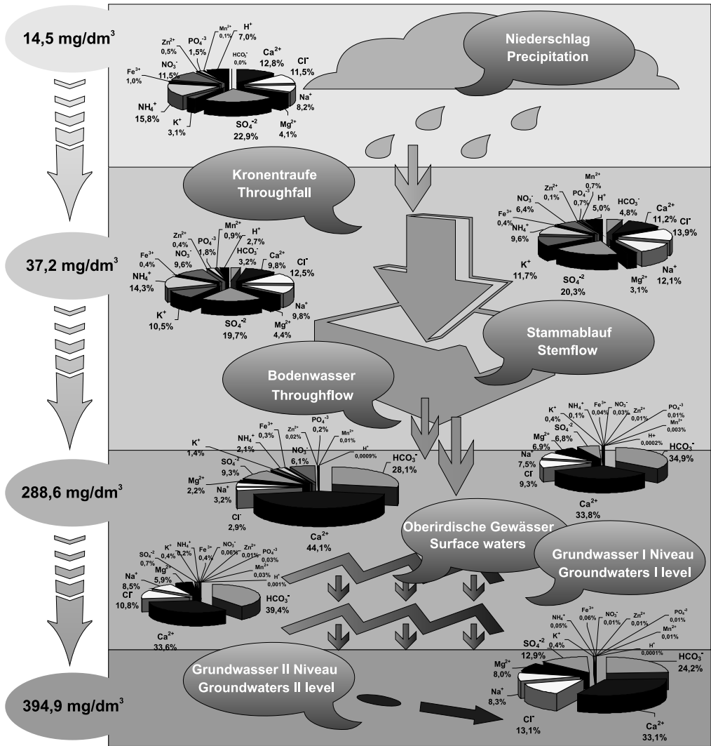
Abb. 9 Wasserkreislauf im Einzugsgebiet des Gardno-Sees. Mineralisation und Ionenanteil für die Jahre 1997 bis 2005.
