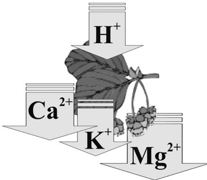
Abb. 6 Ionenaustausch zwischen Niederschlagswasser und Assimilationsorganen.
