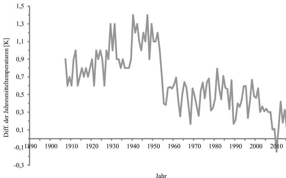
Abb. 7 Differenzen der Jahresmitteltemperaturen zwischen Halle (Saale) und Lindenberg von 1907 bis 2015.
