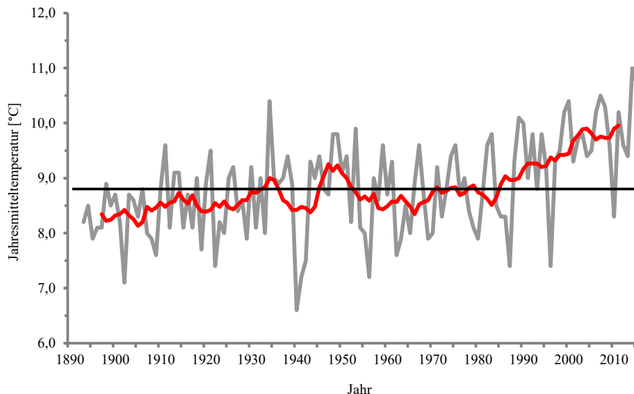
Abb. 3 Jahresmitteltemperaturen (graue Linie) sowie der 9-jährige gleitende Durchschnitt (rote Linie) und der Mittelwert (horizontale Linie) für 1893 bis 2015 für Potsdam. Quelle: DWD 2016.
