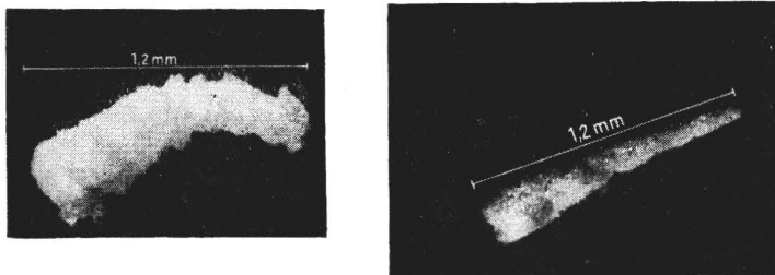
Abb. 11. Tentaculitenreste aus sedimentären Kalklagen, 1. Straßenbiegung hinter den Pferdeköpfen in Richtung Grillenberg
