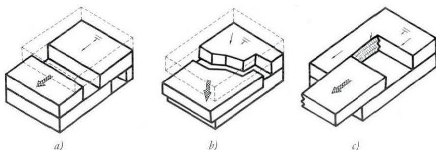
Abb. 2: Bildung tektonischer Großräume durch lokales Zerreißen von Schichtpaketen. a und b: Geradliniger und mehrfach winkelter Raumverlauf; c: Entstehung der steil einfallenden und in der Bewegungsrichtung streichenden Verwerfungsflächen mit Horizontalstriemung, welche die zerrissenen Schichtpakete von denen, die der Zerrung standgehalten haben, abgrenzen (Entwurf: E. Arnberger).
