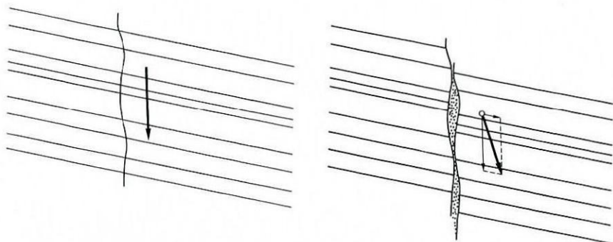
Abb. 3: Entstehung von hohen, schmalen Klusträumen durch Vertikalbewegung entlang schwach-gewellter Bruchflächen (Entwurf: E. Zirkl).
