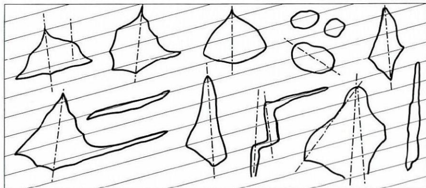
Abb. 1: Auswahl von Raumprofiltypen in der Dachstein-Mammuthöhle. Stark vereinfacht und schematisch gezeichnet. Strichpunktierte Linien geben die an der Raumgestaltung beteiligten Verwerfungen an (Entwurf: E. Arnberger).
