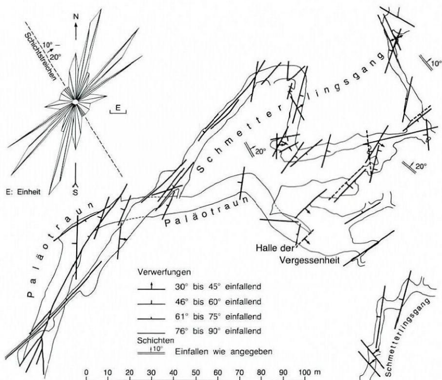
Abb. 5: Streichen und Fallen der Verwerfungen und Schichten im Schmetterlingsgang und in der Paläotraun der Dachstein-Mammuthöhle (Einmessung: E. Arnberger und E. Zirk). Kluftdiagramm: Darstellung des Streichens der Klüfte. Die nördliche Fortsetzung des Schmetterlingsganges ist in der Abbildung rechts unten eingezeichnet.
