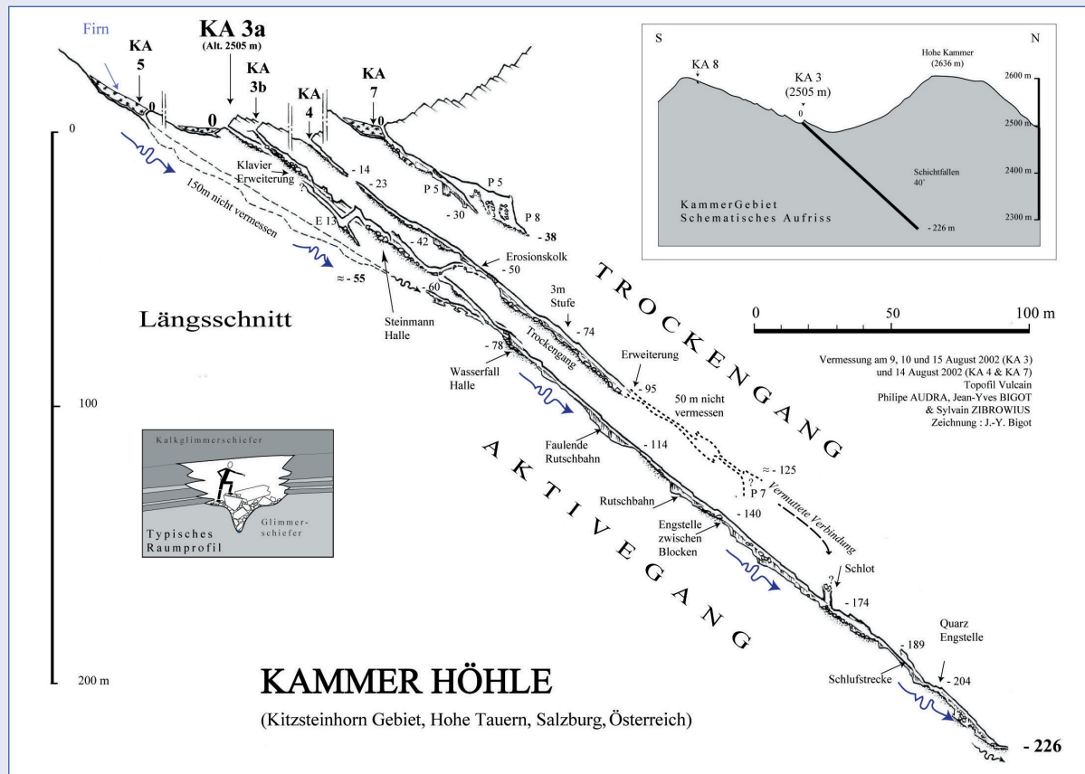
Fig. 6. Cross section of the Kammerhöhle.
