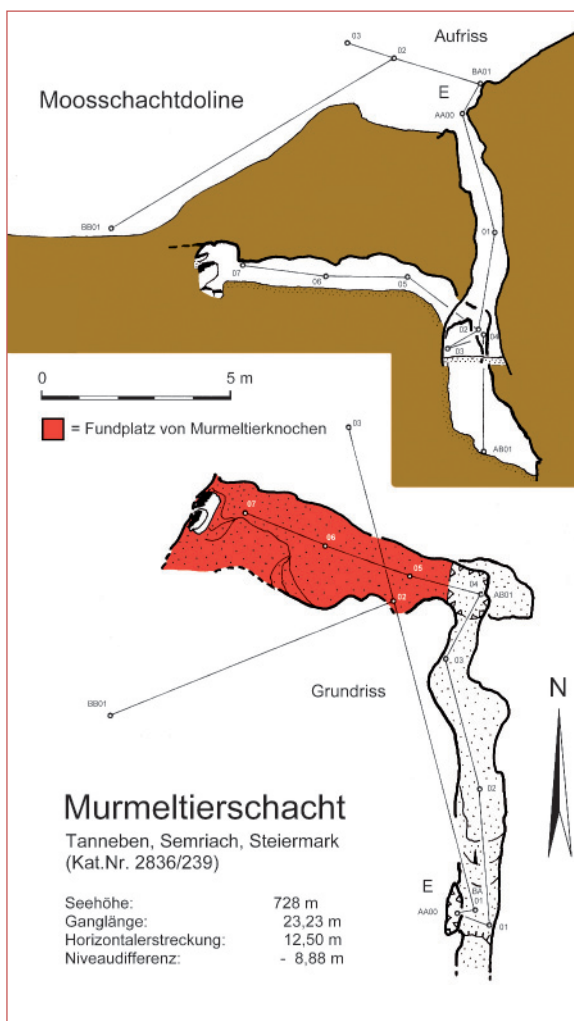
Abb. 4: Höhlenplan, Vermessung: H. Kusch und I. Kusch (12.6.2005), H. Kusch und M. Messner (4.10.2005), Zeichnung: Heinrich Kusch (2006).
