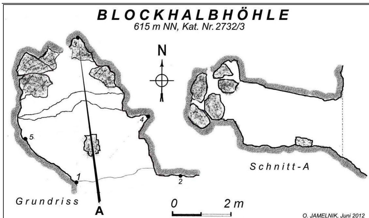
Abb. 2: Blockhalbhöhle - Plan.
