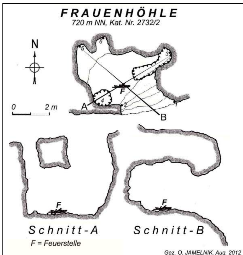
Abb. 1: Frauenhöhle - Plan.
