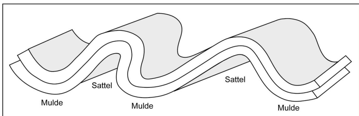
Abb. 1: Schematische Skizze zur inneren Struktur eines gefalteten Gebirges mit Sätteln und Mulden (T. KASIELKE).
