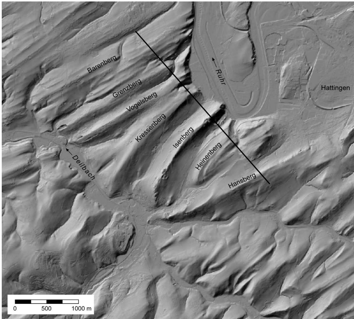
Abb. 2: Geländemodell des Exkursionsbereiches und seiner näheren Umgebung. Die schwarze Linie markiert den Verlauf des in Abb. 3 dargestellten Profils (T. KASSELKE, Kartengrundlage: TIM-online NRW, mit Genehmigung der Bezirksregierung Köln).
