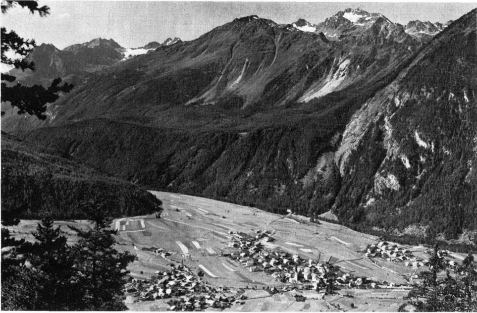
Abb. 3 Umhausen (1036 m), Blick nach Südwest, dahinter Bergsturzgebiet von Kölfels und der Wurzburg. Fast in Bildmitte ein helles Wiesenstück von Kölfels (Standort von Abb. 4).
