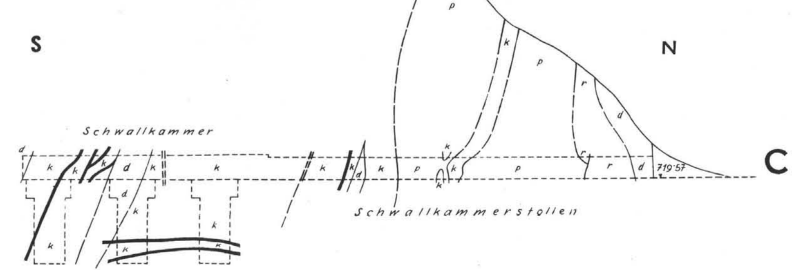
PROFIL: SCHWALKKAMMER UND -STOLLEN (WESTULME) 1:500
