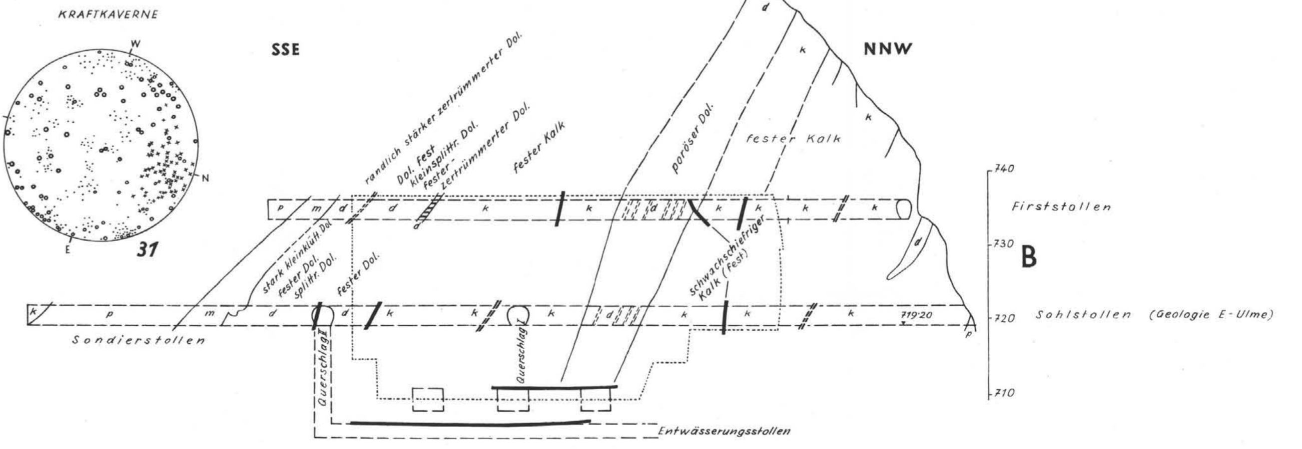
LÄNGSSCHNITT DURCH DIE KAVERNE 1:500
