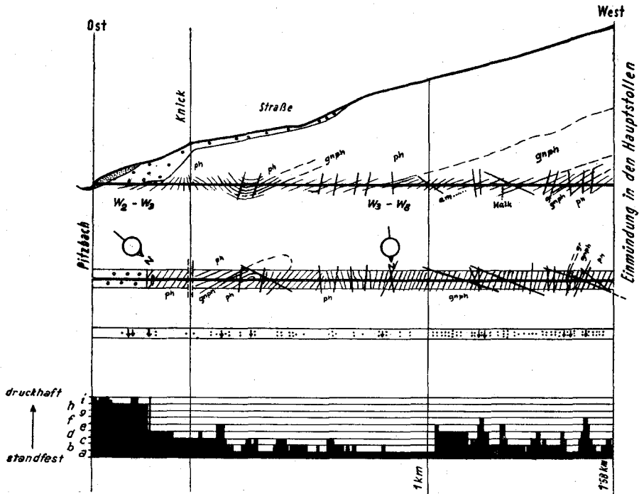
Abb. 2: Längsschnitt durch den Fensterstollen. Geologische Verhältnisse vereinfacht nach der Stollenaufnahme von A. FUCHS.
