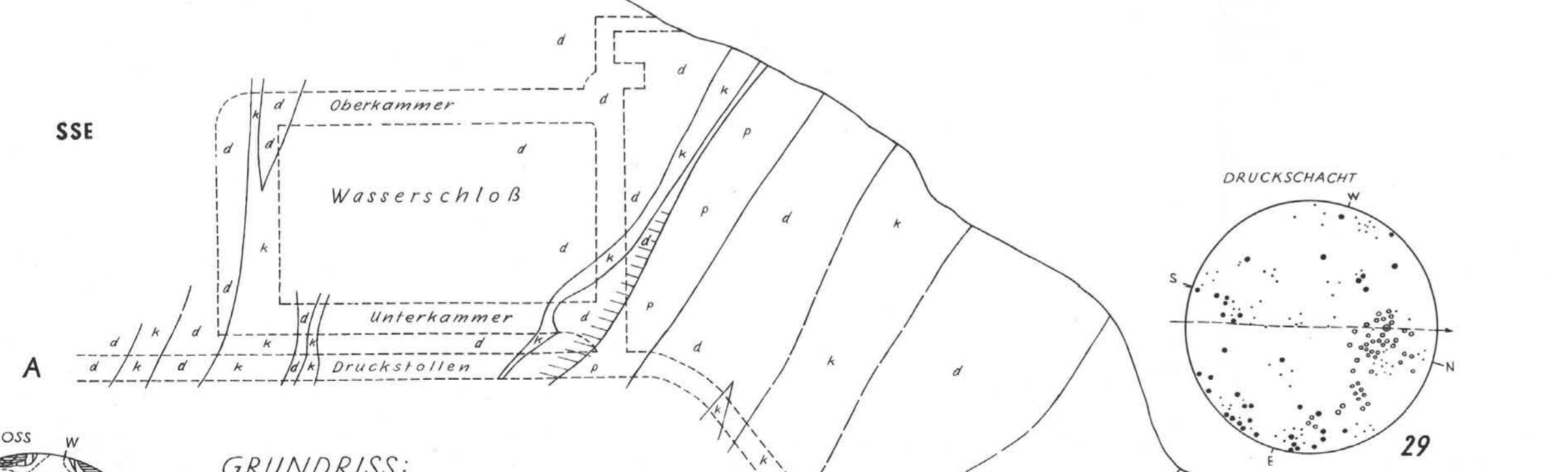
PROFIL: WASSERSCHLOSS-DRUCKSCHACHT 1:1000
