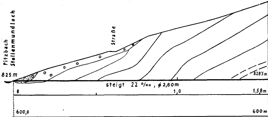
Abb. 1: Geologische Voraussage für den Fensterstollen (Längsschnitt).
