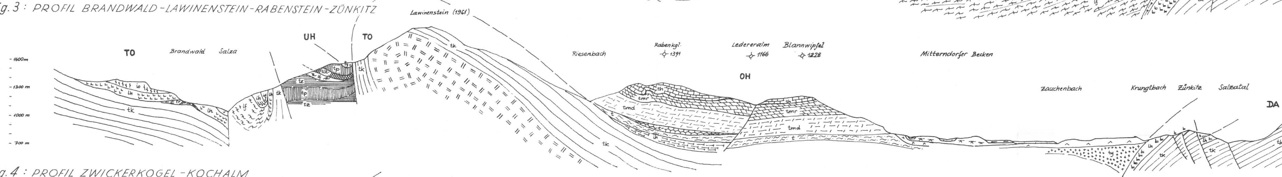
Fig. 3: PROFIL BRANDWALD-LAWINENSTEIN-RABENSTEIN-ZÜNKITZ
