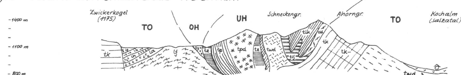
Fig. 5: PROFIL WIENERN-GRASBERG-ALPENGRABEN
