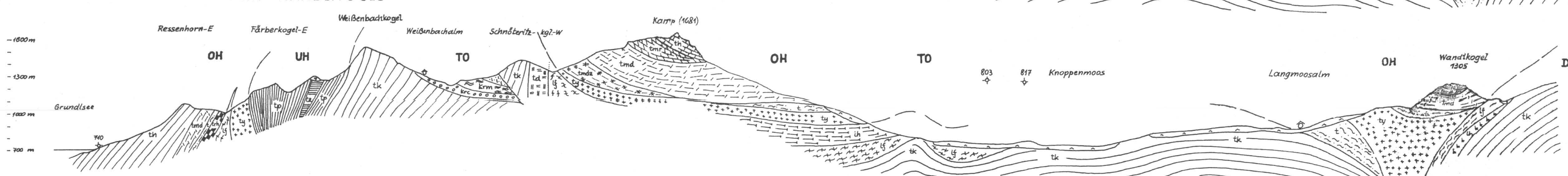
Fig. 7: PROFIL GRUNDLSEE-RÖTHELSTEIN-KAINISCH
