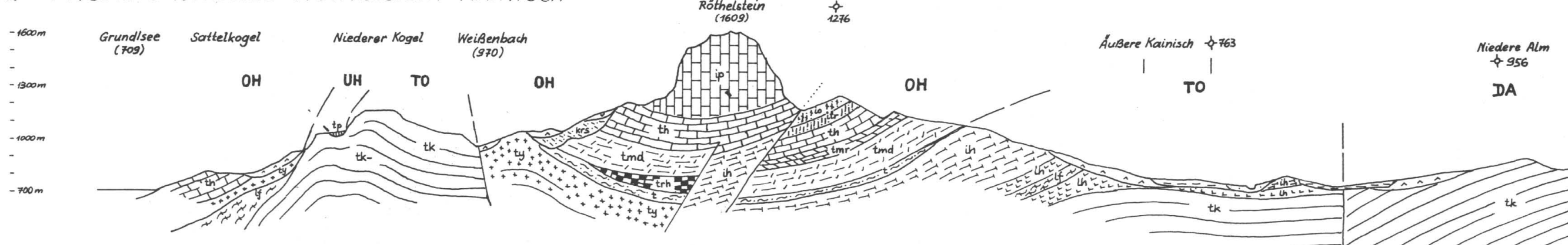
Fig. 7: PROFIL GRUNDLSEE-RÖTHELSTEIN-KAINISCH
