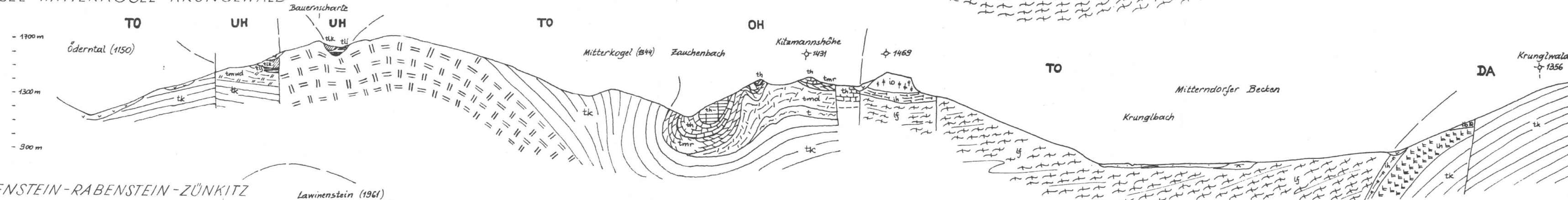
Fig. 2: PROFIL ÖDERNTAL-KRALLERSEE-MITTERKOGEL-KRUNGLWALD
