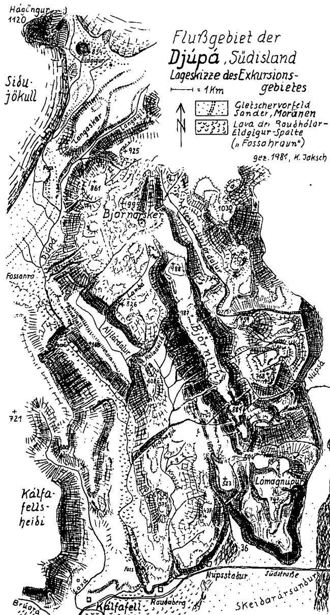
Abb. 1: Flußgebiet der Djúpá, Südisland; Lageskizze des Exkursionsgebietes.
