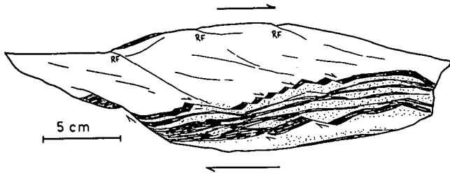
Abb. 10: Schleppung und Zerschierung von Ultramylonit (schwarz) in Biotit-Plagioklas-Gneis. Punktiert: hellgrüner Mylonit bis Ultramylonit. RF = Riedel'sche Flächen. Handstück St 7/20.
