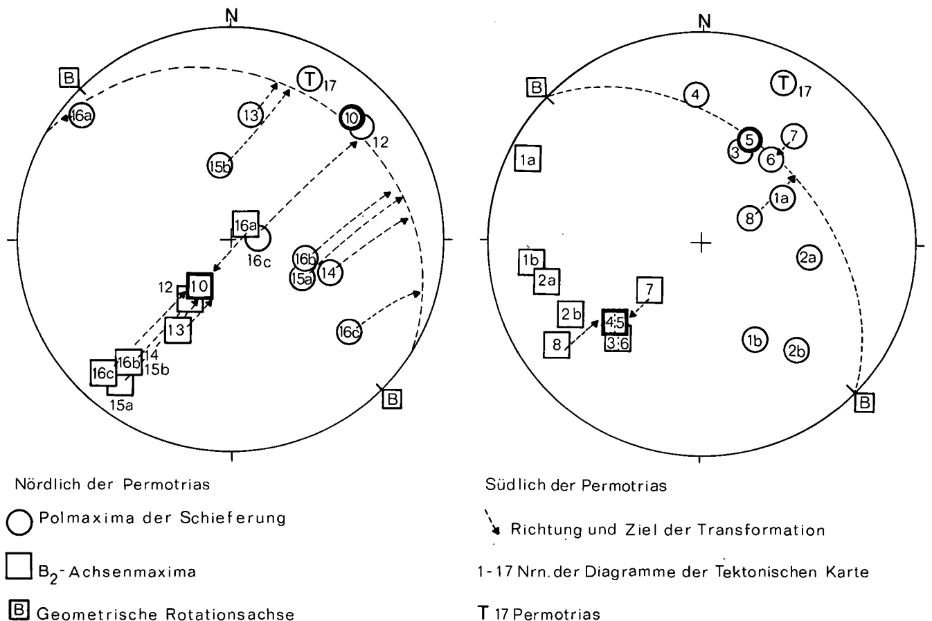
Abb. 13: Sammeldiagramme zur Tektonik des Altkristallins nördlich und südlich der Permotrias.
