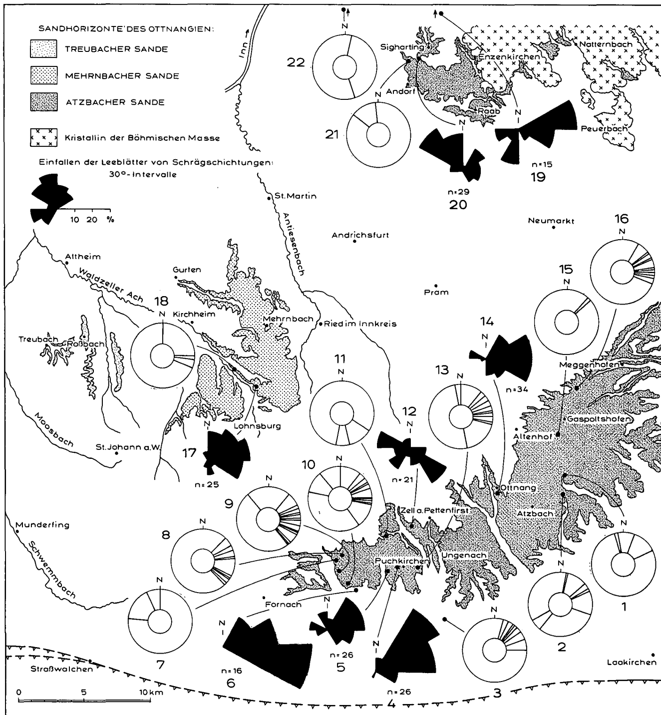
Abb. 27. Paläoströmungsdaten aus Sandhorizonten des Ottnangiens. Geologische Kartengrundlage von F. ABERER (1958). Atzbacher Sande und Übergangsbereich zu Vöcklaschichten: 1 = Aufschlußgruppe um Wufing, ca. 3 km NE Atzbach; 2 = Sandgrube Kasberg; 3 = Sandgrube Timelkam; 4 = Sandgrube Puchkirchen-Berg; 5 = Aufschlußgruppe um Neukirchen/Vöckla; 6 = Aufschlußgruppe an der Vöckla, E Zipf; 7 = Sandgrube Haslau; 8 = Bachaufschluß Haslau-Neue Welt; 9 = Aufschluß bei Brauerei Zipf; 10 = Aufschluß S Brauerei Zipf; 11 = Aufschlußgruppe um Wirtshaus in der Röd, ca. 3 km SSW Ampflwang; 12 = Sandgrube Bruck, SSE Ampflwang; 13 = Sandgrube Roith; 14 = Sandgrube Ottnang-Fischer; 15 = Aufschluß bei Obelstham; 16 = Aufschlüsse bei Hochwasserschutzbauten der Innkreisautobahn A8, N Gaspoltshofen. Mehrnbacher Sande: 17 = Sandgrube Magetsham; 18 = Aufschluß SE Rödham. Enzenkirchner Sande und Fossilreiche Grobsande: 19 = Sandgrube N Mitterndorf; 20 = Sandgrube Seifriedsedt; 21 = Aufschluß an der Pram, N Andorf; 22 = Sandgrube NNE Höbmansbach.
