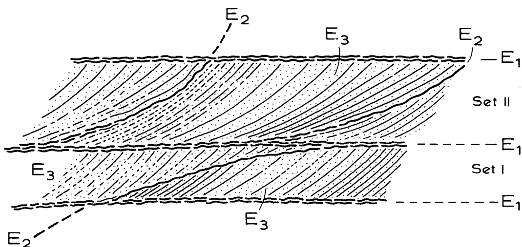
Abb. 6. Schematische Darstellung des Schrägschichtungstyps von Sandwellen der Lithofazies A 3 -A 4 und B 1 -B 2 . Hierarchie der Flächen im Sinne von J. R. L. ALLEN (1980).
