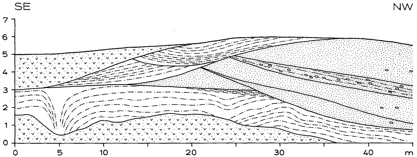
Abb. 2. Atzbacher Sande. Schematische Darstellung eines Großaufschlusses beim Bau der Innkreisautobahn A8 bei Meggenhofen. Erosive Rinnensande mit Pelitklasten der Lithofazies A 1 (Punktsignatur), Feinsand-Mergel-Wechsellagerung mit Entwässerungsstrukturen der Lithofazies C 1 (Strich-Punkt-Signatur), Schuttbedeckung (Häkchensignatur).
