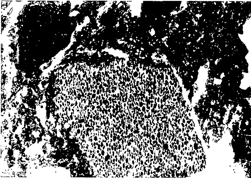
Abb. 14. Reichenhaller Brekzie vom Fuß der Steinbergwand im Halltal. Dicht gepackte Pelmikritklasten bilden die Hauptmasse der Komponenten. Probe Nr. 76; Bildbreite = 17 mm.
