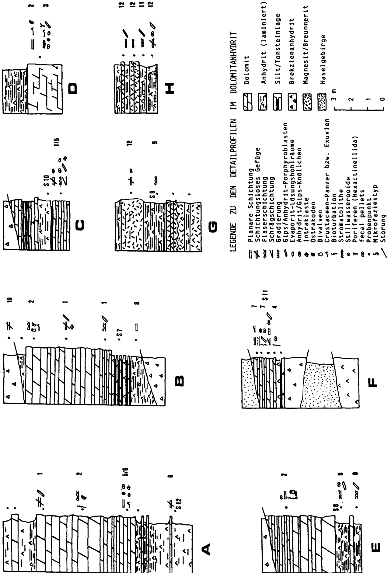
Abb. 4. Detailprofile aus dem Dolomitanhydrit-Komplex der Reichenhaller Schichten des Haller Salzberges. Die Lage der Profile ist aus Abb. 3 ersichtlich; die S-Nummern beziehen sich auf die S-Isotopenproben.
