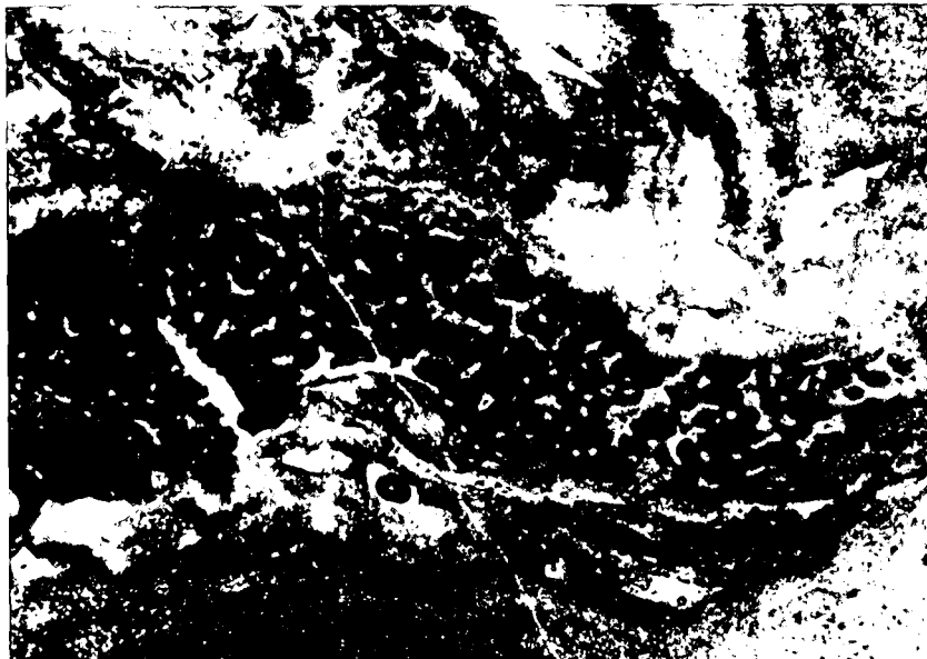
Abb. 9. Auf einer Stromatolithlage aufgewachsener hexactinellider Schwamm. Probe KÖ 1c; Bildbreite 9,3 mm.
