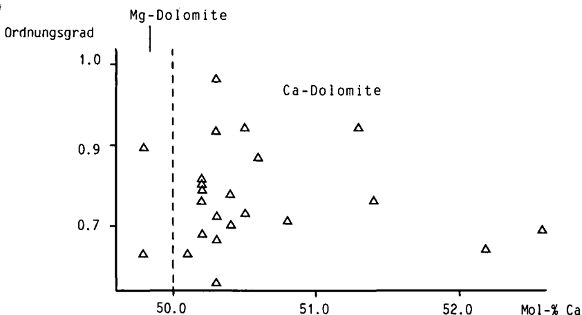
Abb. 16. Streubereich der Ca-Gehalte und Ordnungsgrade der untersuchten Dolomite.
