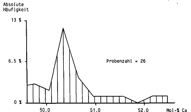
Abb. 15. Histogramm-Darstellung des Ca-Gehaltes der Dolomite.
