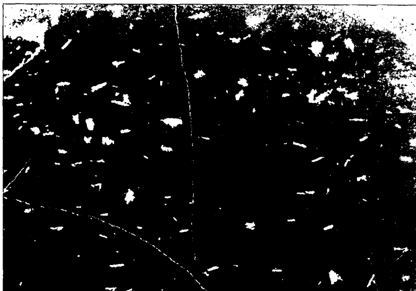
Abb. 6. Fossilfreier, feingeschichteter Dolomikrit mit Lösungshohlräumen von Gips-Kristallen. MFT 1; Probe KA1 14; Bildbreite = 17 mm.
