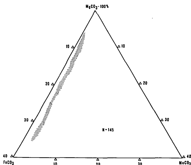
Abb. 17. Teilausschnitt aus dem Dreiecksdiagramm Magnesit – Siderit – Rhodochrosit mit Lage der Proben des Haller Salzberges.
