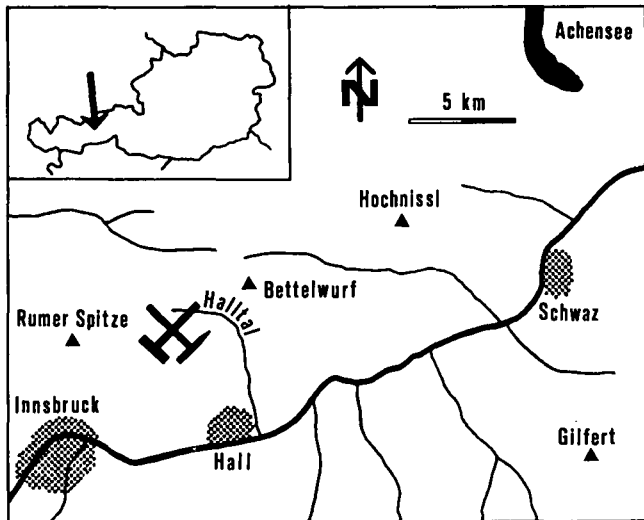
Abb. 1. Lage des Untersuchungsgebietes: Der 1967 stillgelegte alpine Salzbergbau im oberen Halltal.
