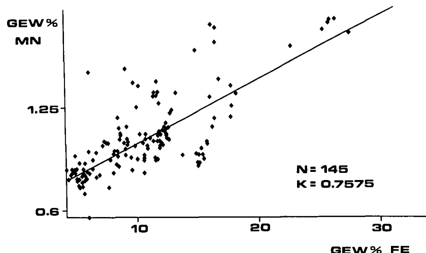
Abb. 18. Lineare Korrelation Fe/Mn von Haller Breunneriten.
