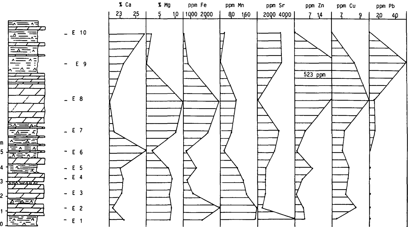
Abb. 20. Detailprofil I (siehe Abb. 3) aus dem Dolomitanhydrit-Komplex des Erzherzogsberg-Horizontes mit geochemischer Auswertung.
