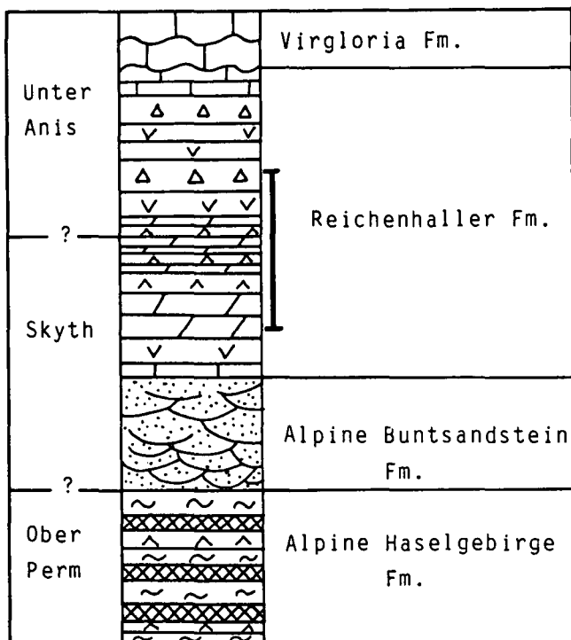
Abb. 2. Stark schematisiertes Übersichtsprofil der basalen permoskythischen Stratigraphie im Untersuchungsgebiet der westlichen Nördlichen Kalkalpen. Der dunkle Balken markiert in etwa das stratigraphische Niveau der untersuchten Dolomitanhydrite.
