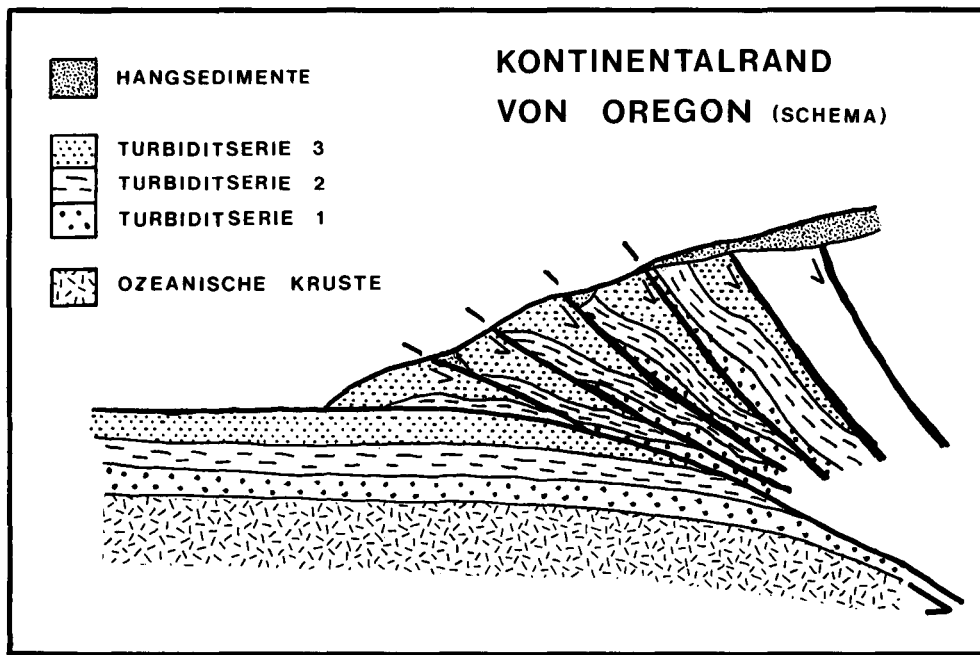
Abb. 4. Schematischer Schnitt durch den Kontinentalrand von Oregon (USA).
