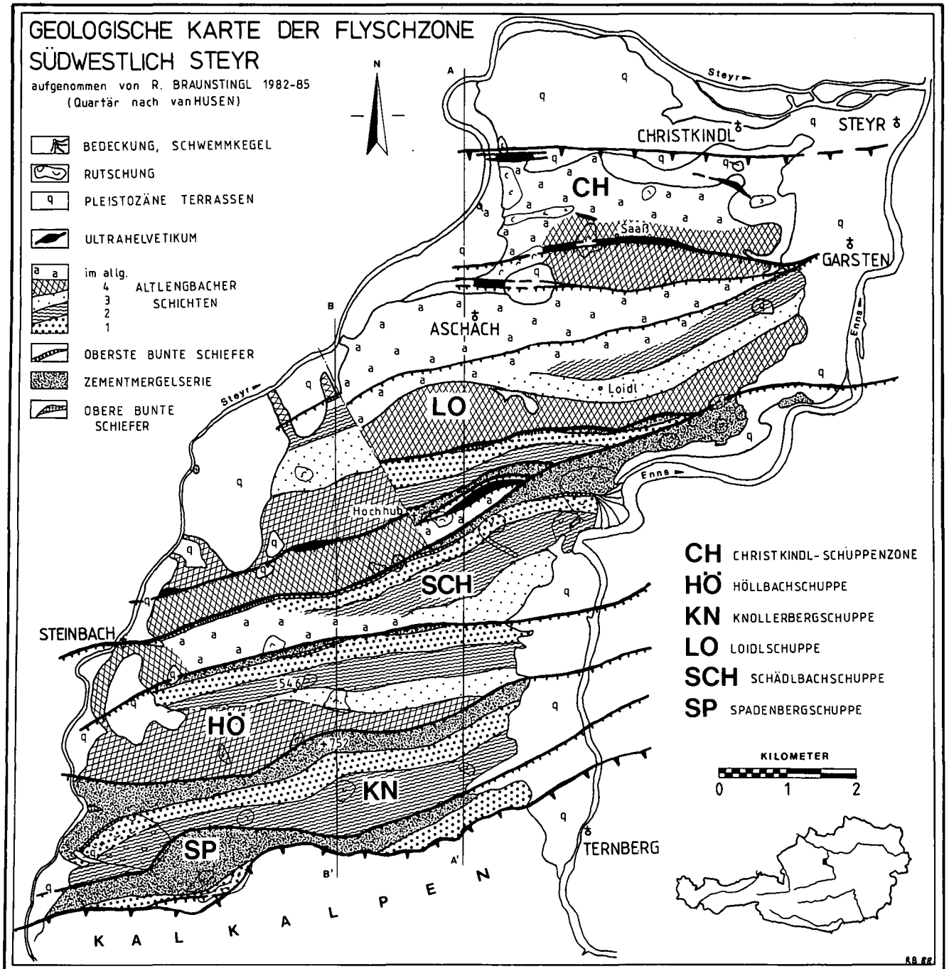
Abb. 2. Geologische Karte der Flyschzone südwestlich von Steyr. Tieferer Flysch (Gaultflysch, Untere Bunte Schiefer, Reischberger Sandstein) ist in diesem Maßstab nicht darstellbar.
