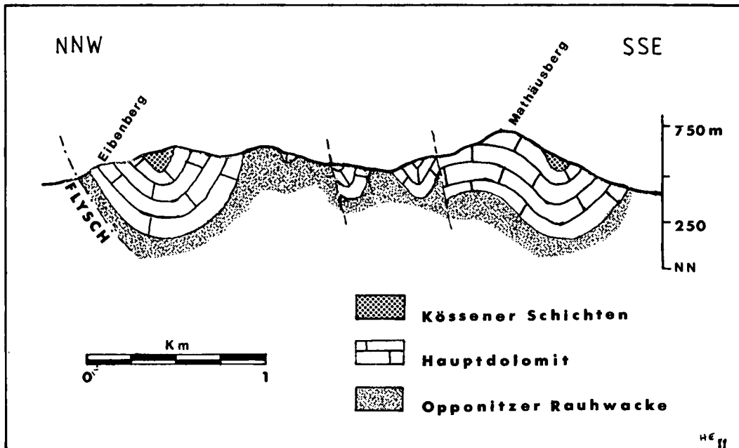
Abb. 3. Profil 2. Der hier ersichtliche einfache Faltenbau ist auch für den Windhagberg und den Mistlberg typisch.
