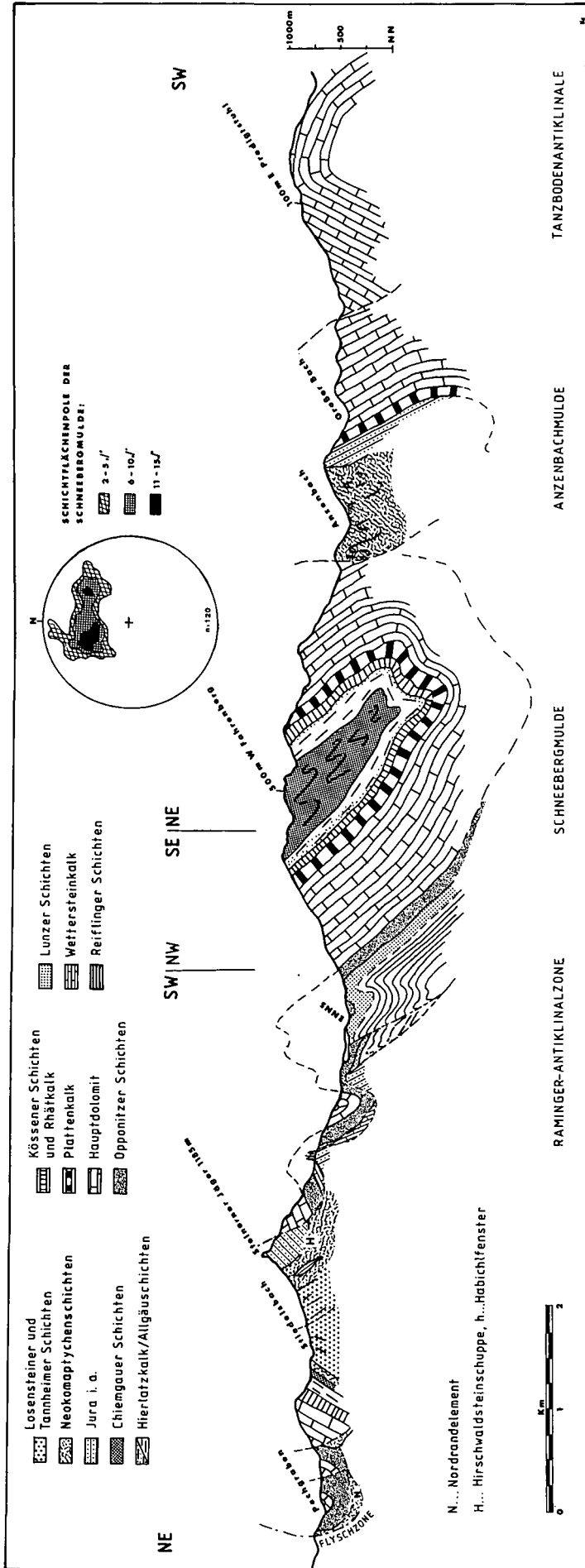
Abb. 2. Profil 1. Deutlich ist die breite, schräg durchsicherte Antiklinalzone im Bereich des Ennstales zu erkennen. Auch gegen Westen schneidet die Basalläche die Schichtfolge schräg an, taucht nach unten und verläuft im Bereich des Dirnzuges in den Reiflinger Schichten. Die Achsen der gezeigten Falten fallen durchwegs in eine östliche Richtung ein.
