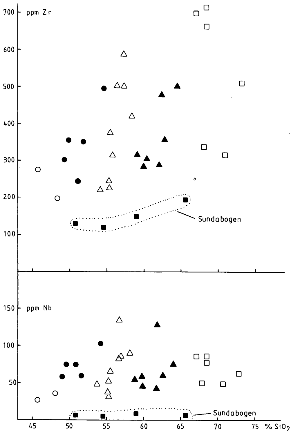
Abb. 4. Zr-Nb- SiO_2 -Diagramm für 29 Analysen von Metavulkaniten aus der südlichen Saualpe. Zum Vergleich ist das Feld von kalkalkalischen Basalten, basaltischen Andesiten, Andesiten und Dazitzen des Sunda-Bogens (WHITFORD et al., 1979) dargestellt (■ umgeben von punktierter Linie). Die Werte sind H_2O - und CO_2 -frei berechnet. Symbole wie auf Abb. 5.
