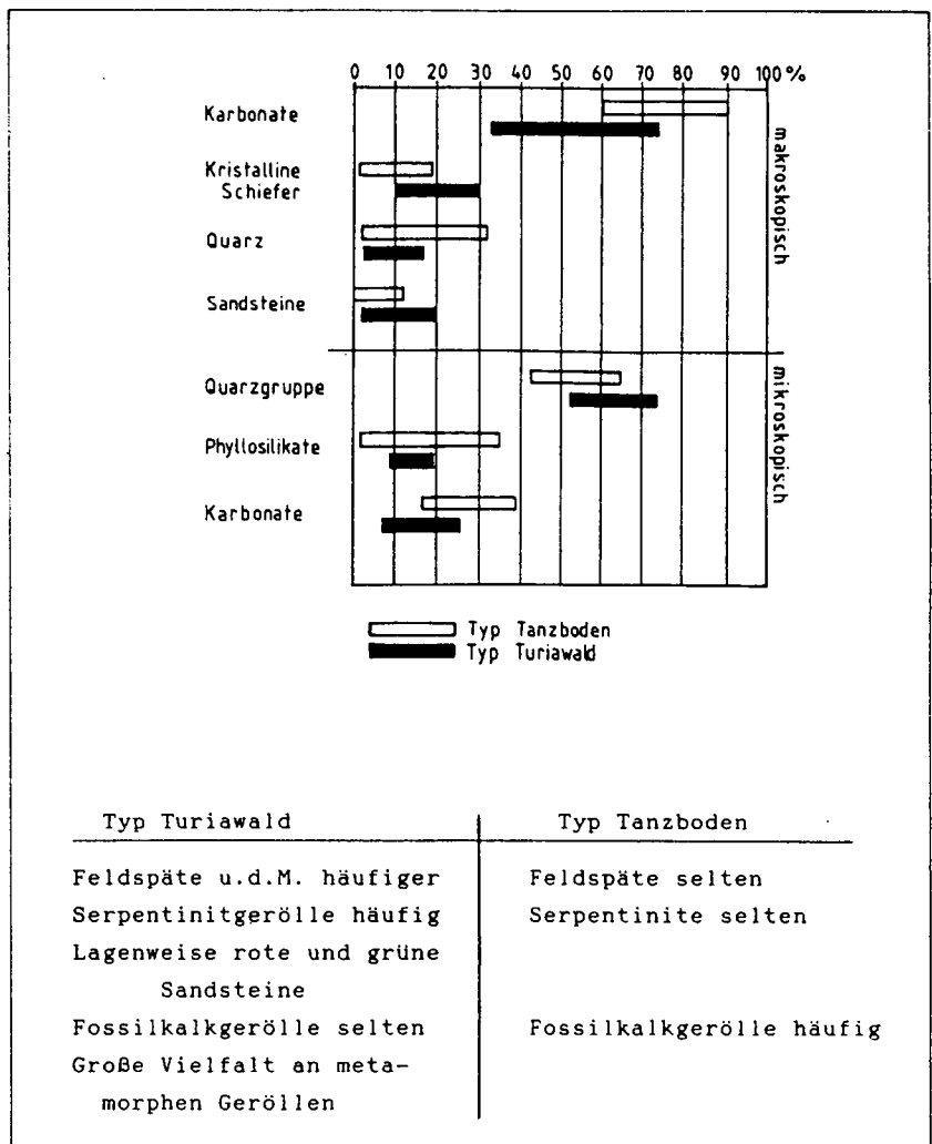
Abb. 6. Statistische Unterscheidungskriterien der Typen „Tanzboden“ und „Turiawald“ des Sattnitzkonglomerates.
