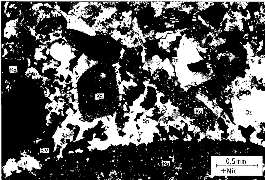
Abb. 5. Dünnschliff des Sattnitzkonglomerates. Ausschnitt aus dem Matrixbereich einer grobklastischen Lage. Die fein- bis mittelsandige Matrix enthält vorwiegend Klaster von Quarz (Qz) neben Karbonat (Ka), Schwermineralien (SM, hier links unten ein Idiomorpher Granat) und Phyllosilikaten (Ph). Im unteren Bildteil grenzt ein großer Karbonatklaster an die Matrix. Das Sediment ist mit Kalzitsparit (Sp) zementiert.
