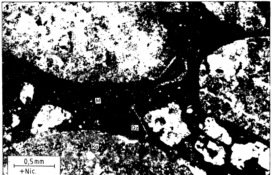
Abb. 8. Dünnschliff des Wellersdorfkonglomerates. Neben den groben, gut gerundeten Karbonatklasten (Ka) treten einzelne subangulare bis angerundete feine Quarzklasten (Qz; Bildmitte mikrokristalliner Quarz) auf. Die kalzitisch zementierte Matrix (M) besteht vorwiegend aus detritischen Dolomitkristallen in Siltfraktion.
