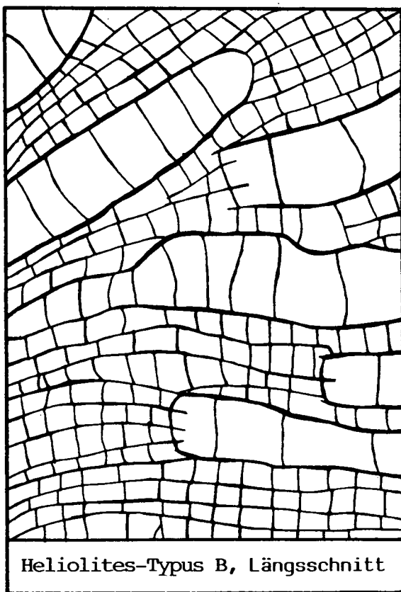
Abb. 3. Darstellung der Heliolites -Morphotypen A, B, C. Vergrößerung 11,5x.
