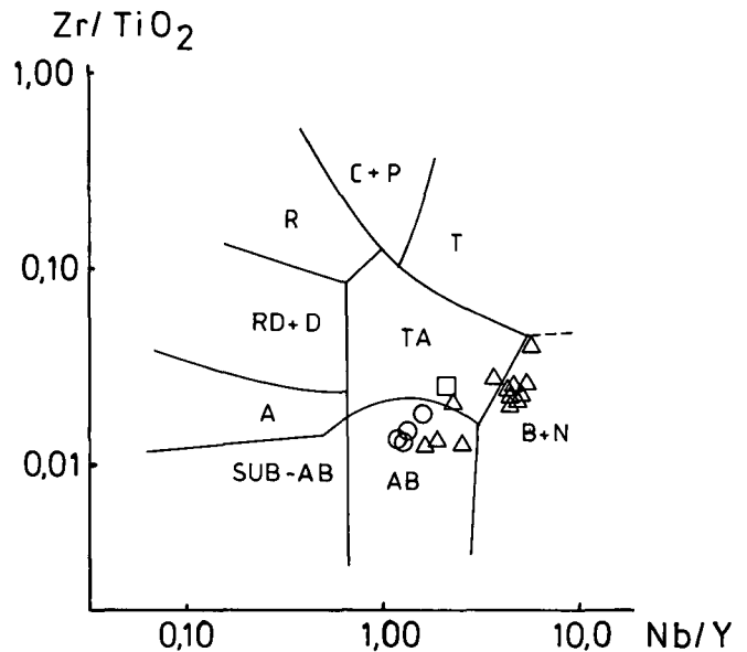
Abb. 7. Zr/TiO_2 -Nb/Y-Diagramm nach FLOYD & WINCHESTER (1978) zur Klassifikation der Eisenhutschiefer. R = Rhyolithe; RD + D = Rhyodazite und Dazite; A = Andesite; SUB-AB = subalkalische Basalte; AB = Alkali-Basalte; TA = Trachyandesite; B + N = Basanite und Nephelinite; T = Trachyte; C + P = Comendite und Pantellerite. Symbole siehe Abb. 5.
