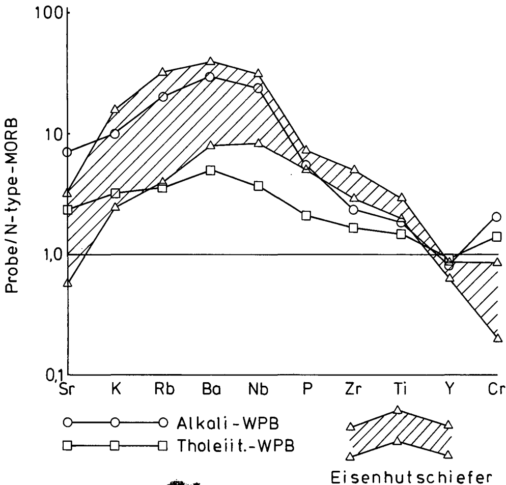
Abb. 8. Ausgewählte Haupt- und Spurenelementgehalte der Eisenhutschiefer normiert mit entsprechenden Gehalten von Basalten mittelozeanischer Rücken (= N-type MORB). Zum Vergleich sind die Werte von Alkali-Intraplattenbasalten (= Alkali-WPB; WPB = „Withinplate Basalt“) und tholeiitischen Intraplattenbasalten (= Tholeiit. WPB) nach PEARCE (1982) mit angegeben.
