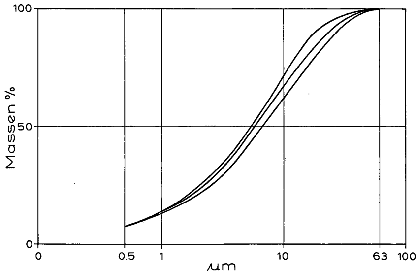
Abb. 12. Kornsummenkurven der abgeseibten Feinfraktion (<0,063 mm) dreier Proben aus den pelitischen Zwischenlagen der Vöcklaschichten. Der Verlauf der drei Kurven ist überaus ähnlich. Der Tonanteil beträgt 20–25 %. Die abgeseibten Feinanteile der Sandproben aus den Vöcklaschichten weisen sehr ähnliche Kornverteilungen auf. Analysiert mit dem Sedigraph 5100 von Micromeritics.
