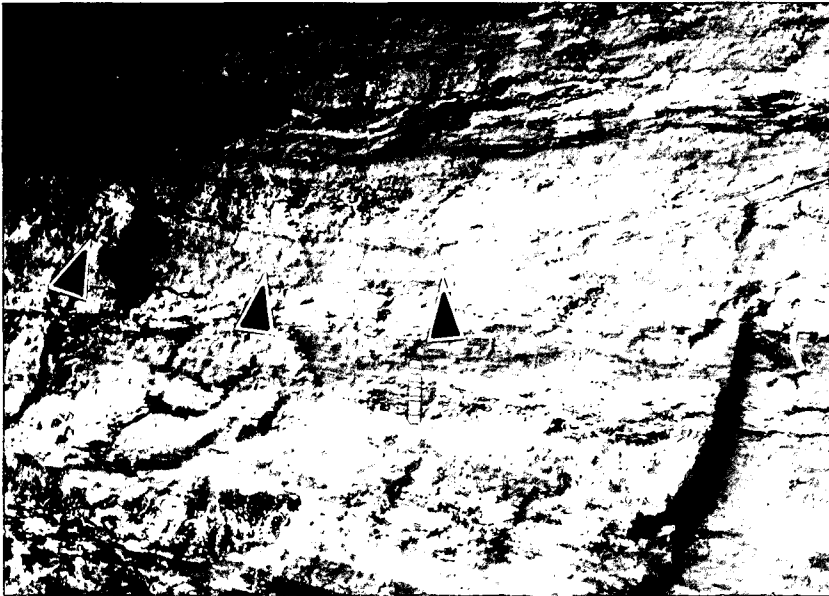
Abb. 4. Lithofazies B 1 und C 2 . Kleine Rinne, 2 m breit, 20 cm tief in einer sandreichen B 1 Einschaltung. Hangend und liegend davon pelitreiches Sediment der Lithofazies C 2 . Vgl. die schematische Darstellung dieser Rinne im Profil Abb. 2 A, bei 5,2 m. Die Rinnenbasis ist deutlich erosiv und pelitisch ausgekleidet; auch in der sandigen Rinnenfüllung finden sich noch pelitische Lagen sowie Pelitklasten. Aufschluß Nr. 19. Länge des Maßstabs: 10 cm.
