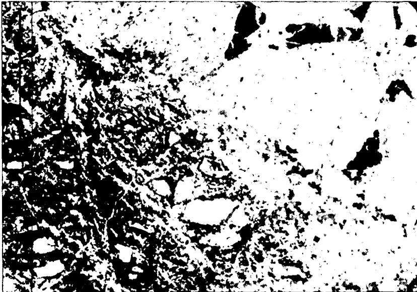
Abb. 2. Gegenüberstellung der beiden Hauptgesteinskomponenten.
