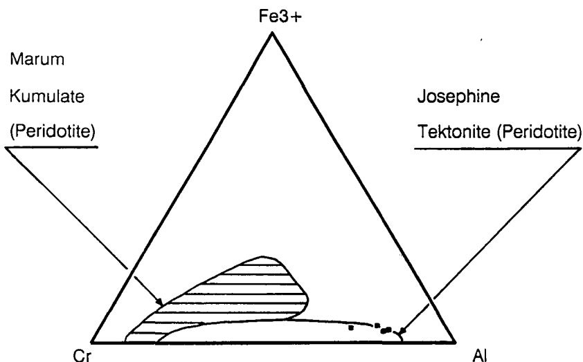
Abb. 10. Dreiecksdarstellung Cr - Fe 3+ - Al zur Unterscheidung von Kumulaten (Marum Peridotit) und Tektoniten (Josephine Peridotit). Symbole wie in Abb. 6.
