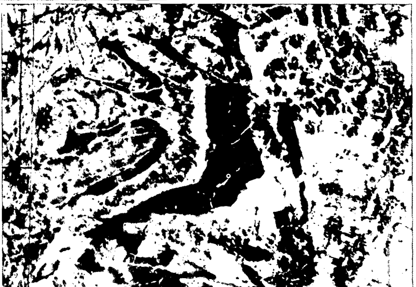
Abb. 3. Spinell, angeordnet in einer Art "Schlingenstruktur" im Bereich einer durch Karbonat und Serpentinmineralen verheilten Kluft. Ein Pol., Bildlänge 3 mm.
