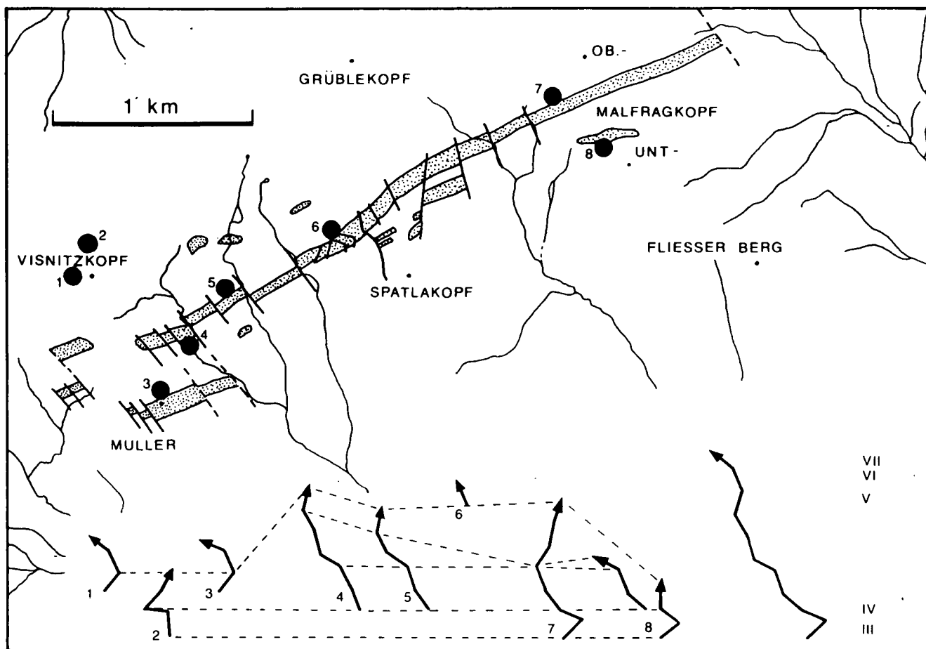
Abb. 4. Ableitung des Bewegungspfad von Schokoladetafeln im Steinsberger Lias (3-8) und in Flysch-Sandsteinen (1+2). Punktiert = Steinsberger Lias. Rechts eine Zusammensetzung der einzelnen Abschnitte mit Numerierung.
