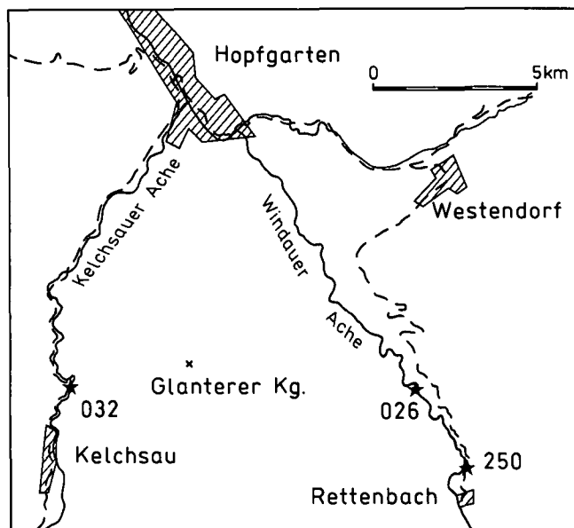
Abb. 2. Detailkarte zur geographischen Lage der Fossilfundpunkte.
