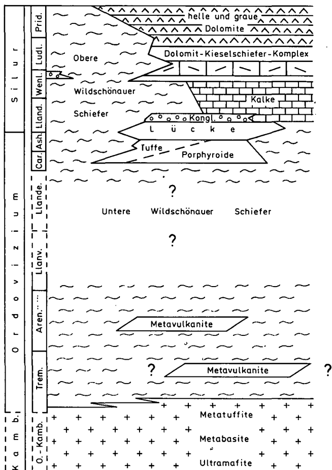
Abb. 3. Faziesschema des prädevonischen Gesteinsinhalts der Nördlichen Grauwackenzone in den Kitzbüheler Alpen. Nach MOSTLER (1983) und mit eigenen Ergänzungen. Prid. = Pridoli; Ludl. = Ludlow; Wenl. = Wenlock; Lland. = Llandovery; Ash. = Ashgill; Car. = Caradoc; Llande. = Llandeilo; Llanv. = Llanvirn; Aren. = Arenig; Trem. = Tremadoc; Kamb. = Kambrium.
