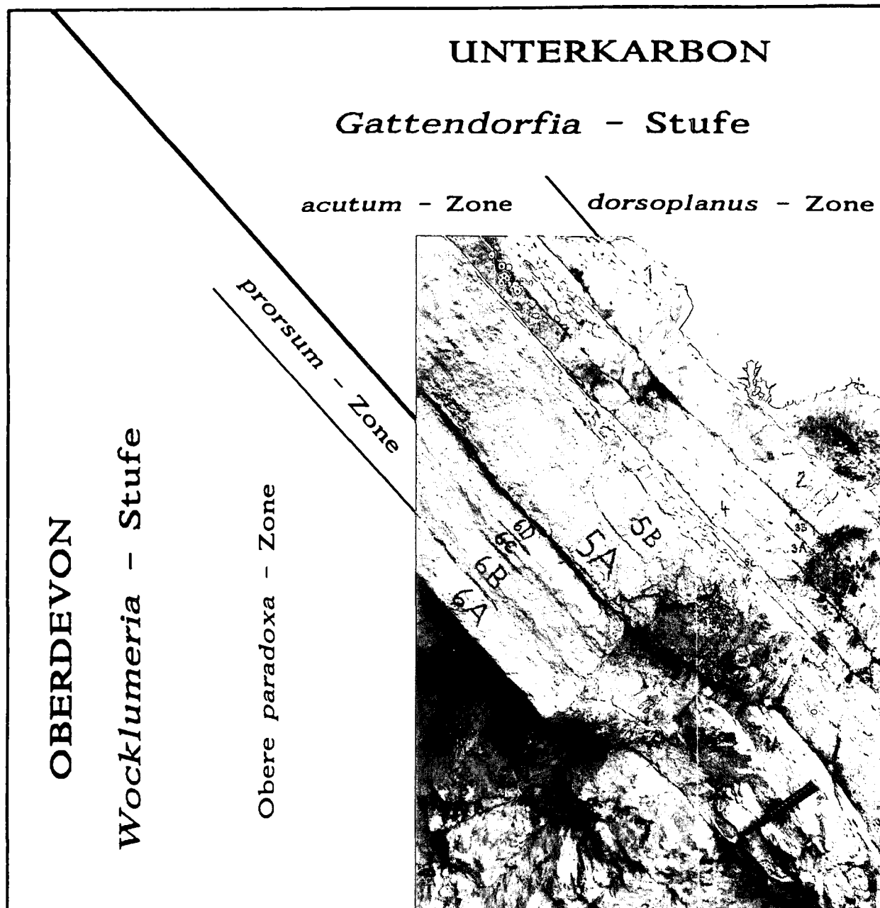
Abb. 2. Devon/Karbon-Grenzbereich des Profiles an der Grünen Schneid. Foto: H.P. SCHÖNLAUB, Juli 1988.
