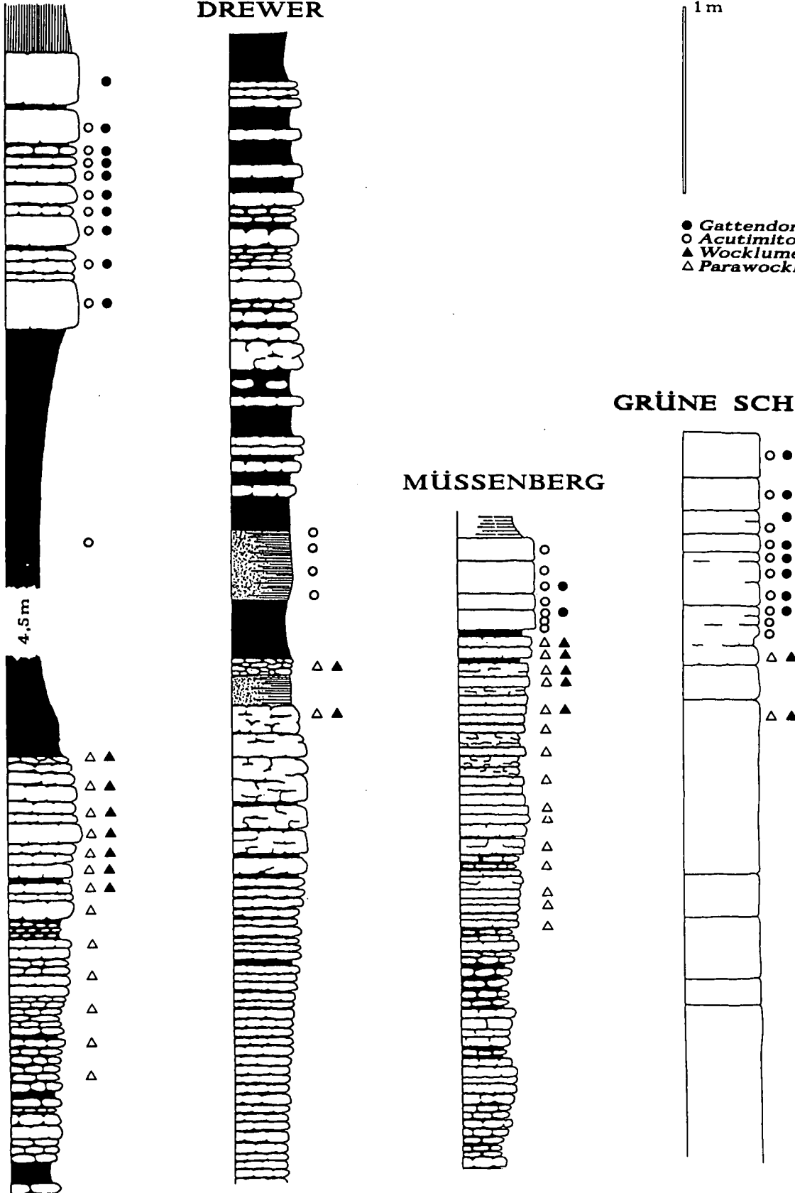
Abb. 5. Korrelation verschiedener Ammonoideen-führender Devon/Karbon-Grenzprofile. Ober-Rödinghausen nach VÖHRINGER (1960), SCHINDEWOLF (1937) und unveröffentlichten Daten. Drewer nach CLAUSEN et al. (1989) und unveröffentlichten Daten. Müssenbergr nach KORN (1981) und CLAUSEN et al. (1990).
