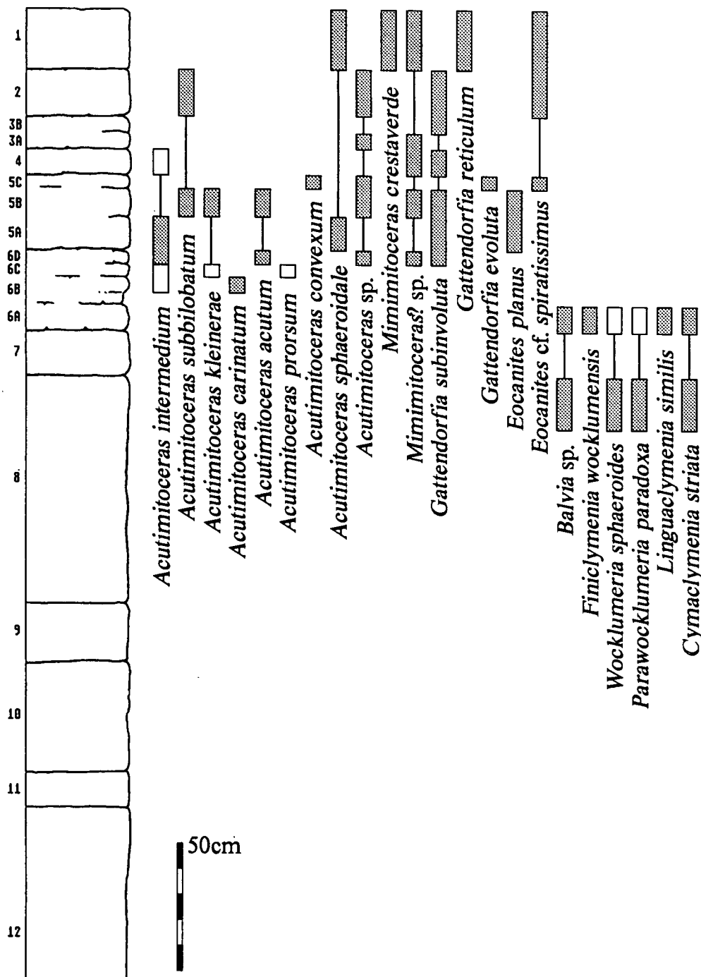
Abb. 3. Schematische Darstellung des Profils mit stratigraphischer Reichweite der gefundenen Ammonoideen.
