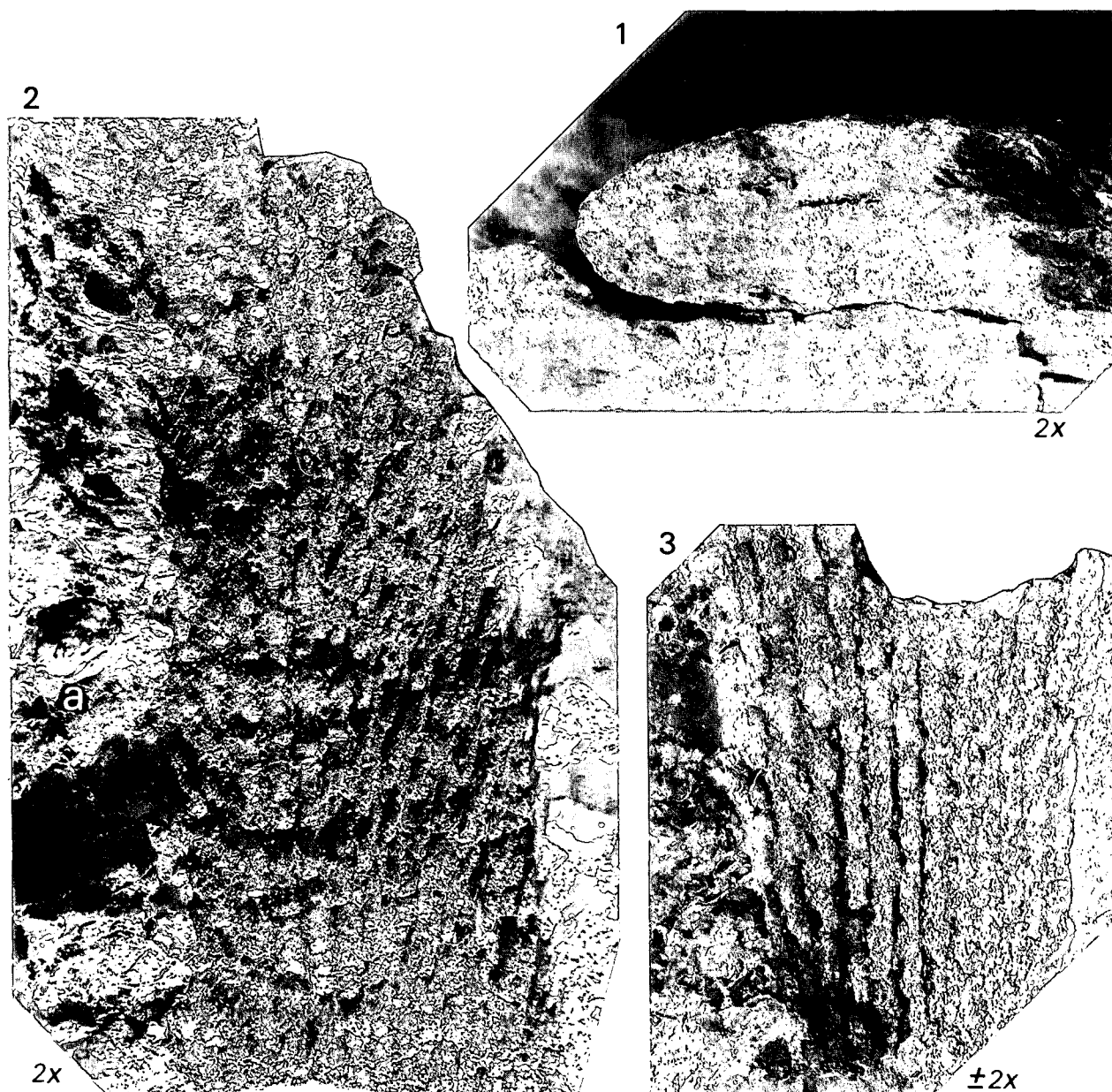
Fig. 1: Knorria sp. Das Stück ist von der Seite aufgenommen. Man sieht einen ovalen Querschnitt des Stammes. Foto Frau Wette (T. H. Aachen), Fotonr. 19. Sammlung Schönlaub im Geol. Bureau Heerlen. Vergr. 2 x.
