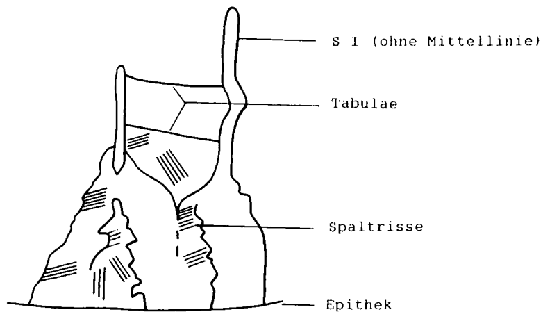
Alaiophyllum
