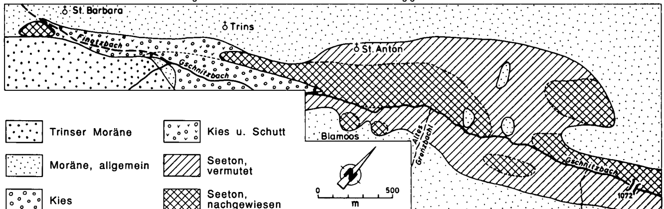
Geologische Kartenskizze des Seetonevorkommens im äußeren Gschnitztal.
