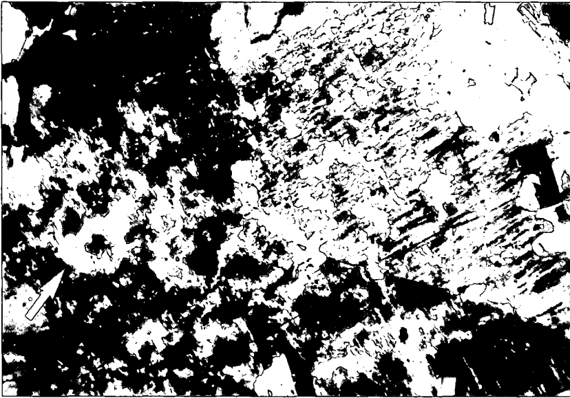
Abb. 3. Großer, nach dem Karlsbader Gesetz verzwilligter Kalifeldspat mit fleckigen und aderförmigen, z.T. verzwilligten (Pfeil) Albitentmischungen. Probe 4, Tristacher Quellbehälter. Länge der unteren Bildkante: 3,2 mm.
