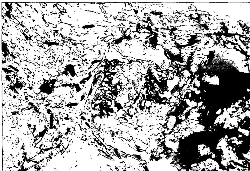
Abb. 5. Im Kern durch Chlorit und Biotit verdrängter Granat. Probe 31, Buchwiese. Länge der unteren Bildkante: 3,2 mm.
