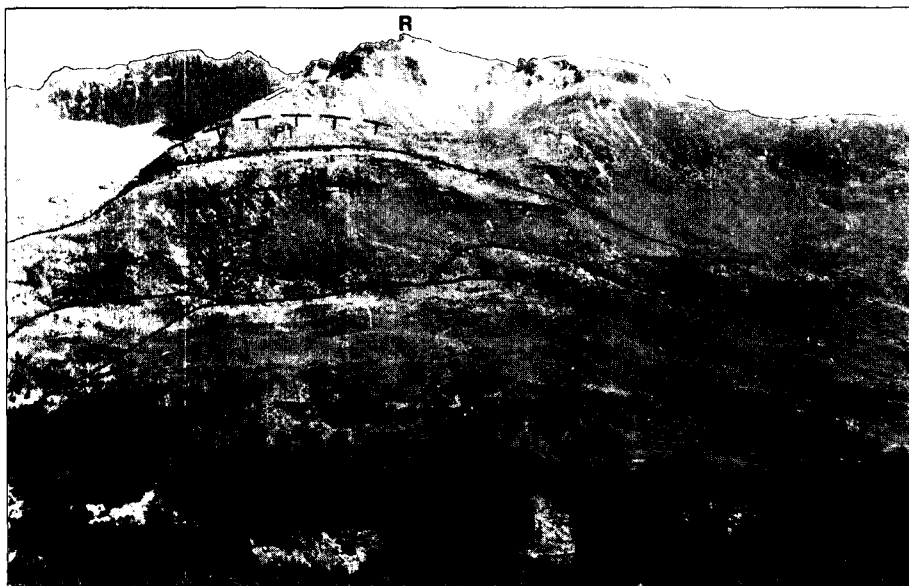
Abb. 1. Zoomgegenhangaufnahme (Standort Feldereralm), aus der die Hauptabrißkanten westlich des Rührkübels (R) und der oberste Bereich des Talzuschubes ersichtlich sind. P1/P2 bezeichnen einen durch schollenförmige Absetzungen versetzten Prasinitzug.
