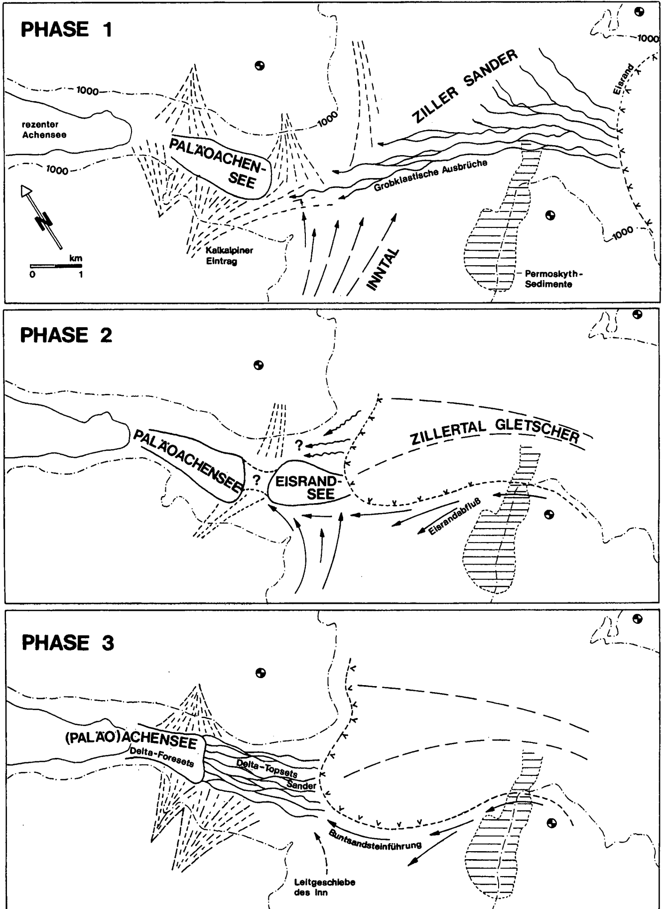
Abb. 7. Entstehung des Achenseedammes; Details zur topographischen Situation siehe Abb. 1.
