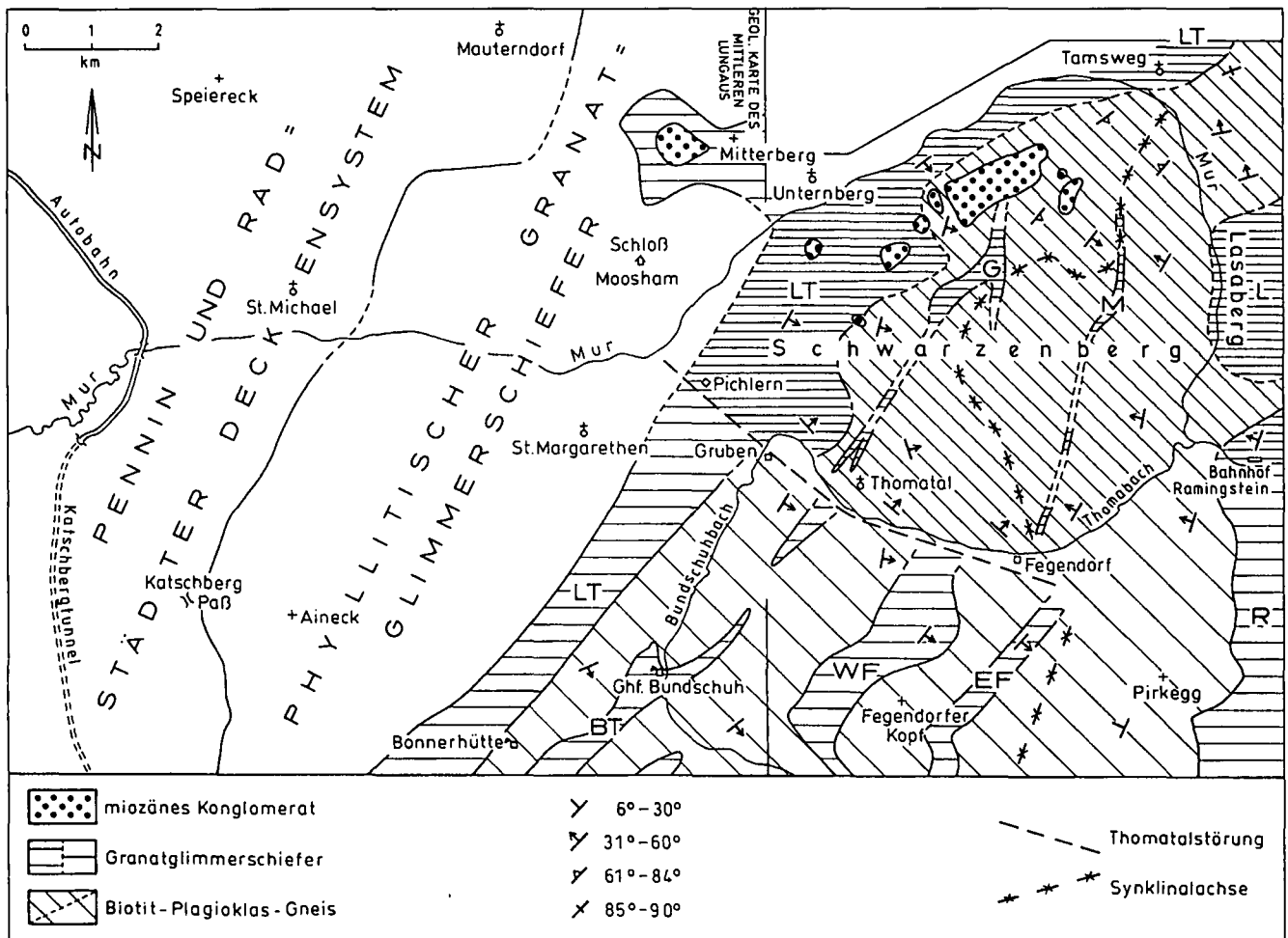
Abb. 3. Tektonische Übersichtskarte des Schwarzenberges bei Tamsweg. Sein Kristallin zeigt eine schüsselförmige Struktur. Der annähernd meridional streichende E-Teil biegt bei Tamsweg nach E. Die Thomatal-Störung läßt eine Diskordanz der s-Flächen erkennen. Das transgressive miozäne Konglomerat bildet den S-Rand des Lungauer Tertiärbeckens und reicht am Mitterberg weit nach W. Nur angedeutet sind die Strukturen der westlichen und südlichen Nachbargebiete des Schwarzenberges. Granatglimmerschieferzüge: LT = Laußnitz-Tamsweg-Zug; BT = Bundschuh-Thomatal-Zug; G = Goldbrunnock-Zug; WF = Westlicher Fegendorfer-Zug; EF = Östlicher Fegendorfer-Zug; M = Maßlhöhe-Zug; R = Ramingsteiner Granatglimmerschiefer und seine Fortsetzung im Halbfenster des Lasaberges (L).
