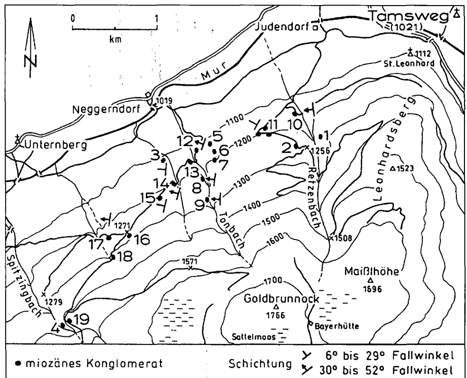
Abb. 4. Kartenskizze der derzeitigen Aufschlüsse des miozänen Konglomerates am Schwarzenberg. Die Nummern entsprechen der Beschreibung der Aufschlüsse in Tabelle 1.
