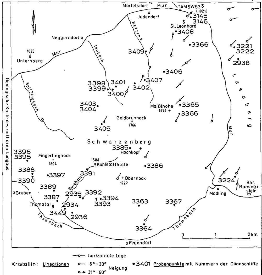
Abb. 1. Lineationen und Probenpunkte im Kristallin des Schwarzenberges. Ergänzung zur geologischen Karte der Abb. 2. Die Dünnschliffnummern sind bei den Probenpunkten angegeben.
