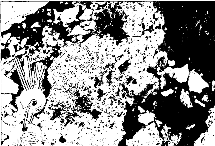
Abb. 4. Bohnerzreiches Feinkonglomerat.
