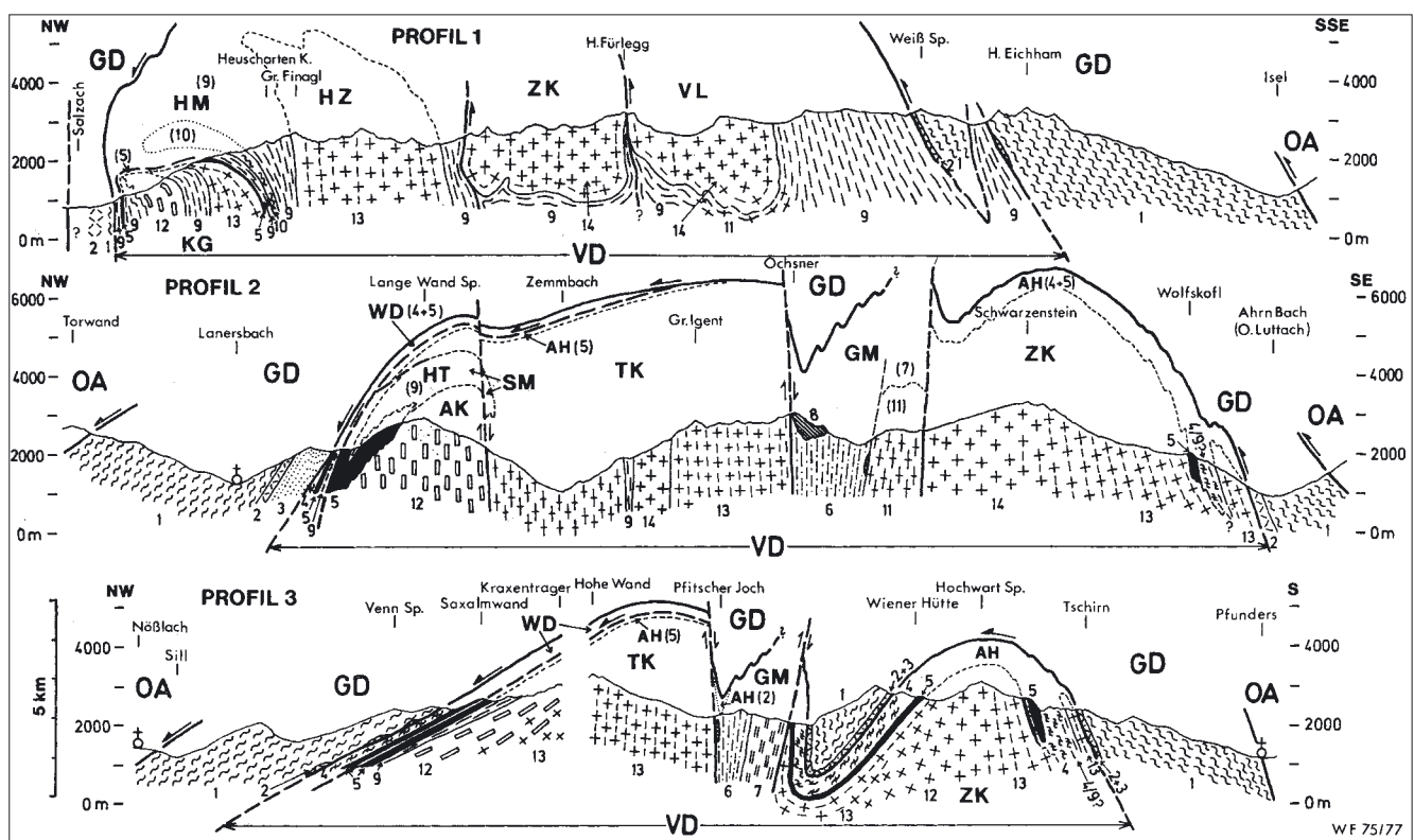
Abb. 3. Profile (nicht überhöht) durch das westliche Tauernfenster, geeignet zur Erläuterung des Problems der zentralen Schieferhülle. Tektonische Begriffe: OA = Ostalpin (undifferenziert); GD = Glocknerdecke; VD = Venedigerdecke, einschließlich KG = Krimmler Gneiswalze; HZ = Habachzunge; ZK = Zillertaler Kern; VL = Venedigerlappen; AK = Ahornkern; TK = Tuxer Kern; HM = Habachmulde; GM = Greiner Mulde; SM = Schönachmulde; HAT = Höllenstein-Tauchdecke; WD = Wolfendordecke; AH = Autochthone Hülle (Mesozoikum). Gesteinsserien: Permomesozoische Hülle: 1 = Bündner Schiefer (Jura–U. Kreide) mit Prasiniten und Serpentiniten; 2 = Triadische Karbonate; 3 = Wustkogelserie (Permoskyth); 4 = Kaserer Serie (U. Kreide); 5 = Hochstegenfolge (Jura). Paläozoische Hülle: 6 = Psephite und Psammite der Greiner Serie (Jungpaläozoikum); 7 = Furtchagschiefer (Graphitbiotitschiefer) (Jungpaläozoikum?); 8 = Serpentin; 9 = Metasedimente und Metavulkanite des Altpaläozoikums (Habachserie), z.T. Altkristallin; 10 = Graphitschiefer in 9 (Habachphyllit). Zentralgneise, Altkristallin: 11 = Migmatite, Anatexite, Bändergneise; 12 = Porphyranitgneis; 13 = Granitoidgneise (Augen-Flasergneis etc.); 14 = Metagranitoid. W. FRISCH (1977; p. 680–681).
