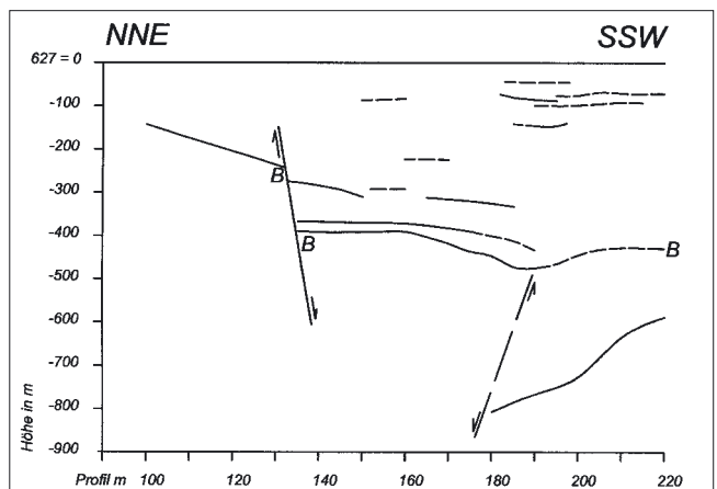
Abb. 7. Tiefenprofil ET 9302 (B = Reflektor der Quartärbasis).
