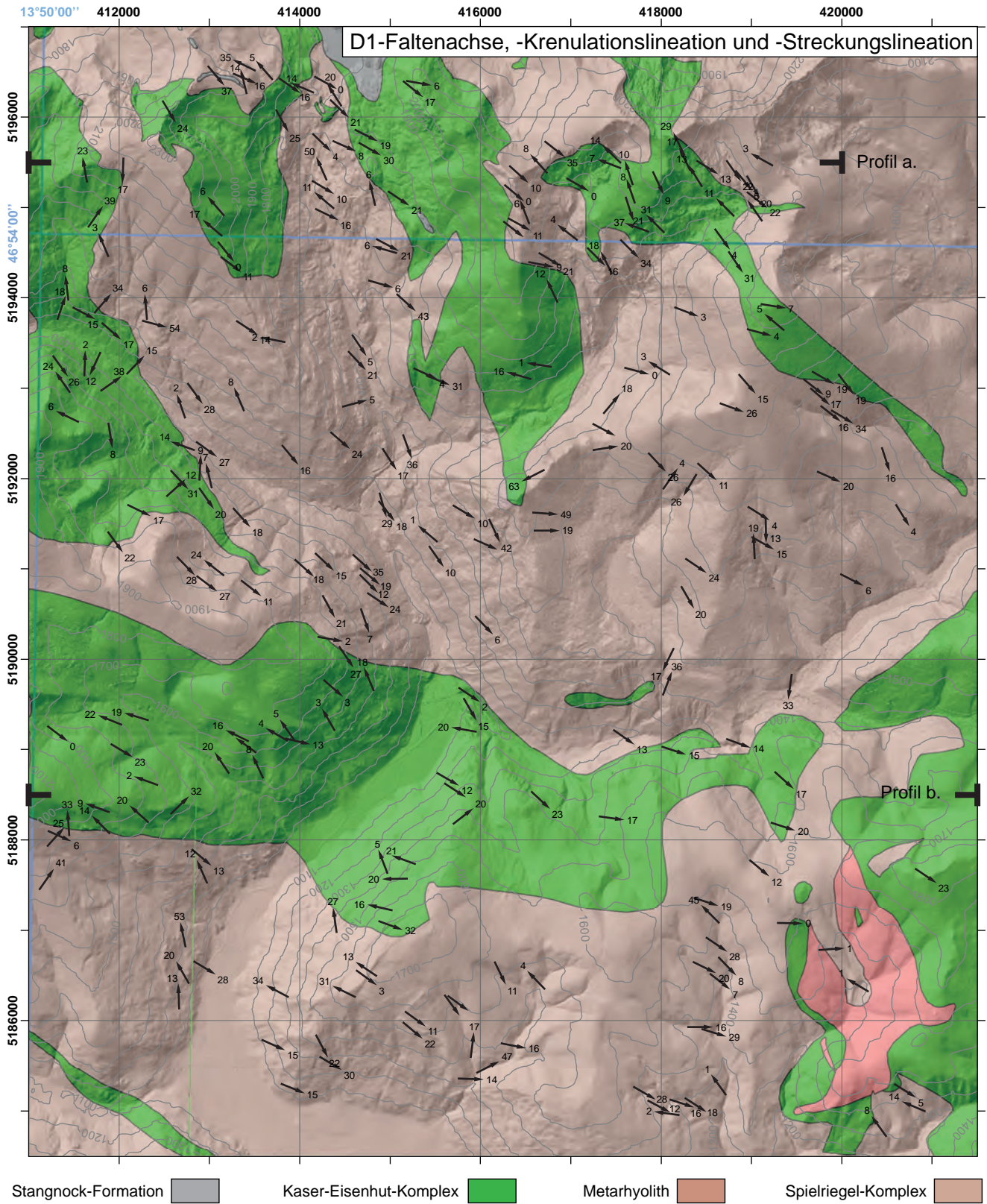
Abb. 7. Karte der D1-Faltenachse, D1-Krenulationslineation und D1-Streckungslineation. Die Nummern bei den Symbolen geben das Abtauchen der Linien an. Aus Gründen der Anschaulichkeit und besseren Lesbarkeit wurde die Anzahl der Symbole reduziert. Abgedeckte geologische Karte im UTM33-Koordinatensystem. Die Isohypsen wurden basierend auf der SRTM-Topografie (FARR et al., 2007) gerechnet. Hillshadekarte aus dem Amt der Kärntner Landesregierung.
