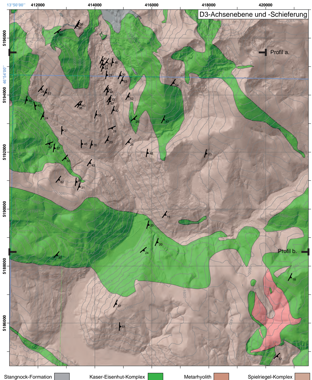
Abb. 10. Karte der D3-Achsebene und D3-Schieferung. Die Nummern bei den Symbolen geben den Fallwinkel an. Aus Gründen der Anschaulichkeit und besserer Lesbarkeit wurde die Anzahl der Symbole reduziert. Abgedeckte geologische Karte im UTM33-Koordinatensystem. Die Isohypsen wurden basierend auf der SRTM-Topografie (FARR et al., 2007) gerechnet. Hillshadekarte aus dem Amt der Kärntner Landesregierung.
