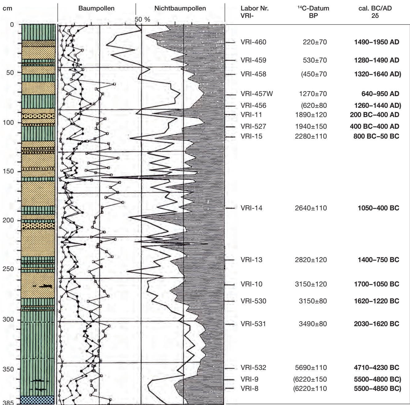
Abb. 4. Stratigraphie, Hauptdiagramm und die Radiokarbondaten im Pollenprofil des Buntten Moores.
