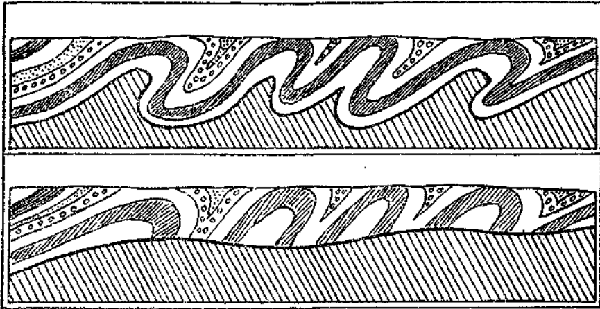
Fig. 11. Das Grundrelief ist schräffelt. Im oberen Fall ist die Schubahn mit der Hangendschubmasse verfaltet, im unteren Fall schneidet die Faltenstruktur der Schubmasse an der Schubahn ab. Nur der untere Fall ist noch weiter schubfähig.
