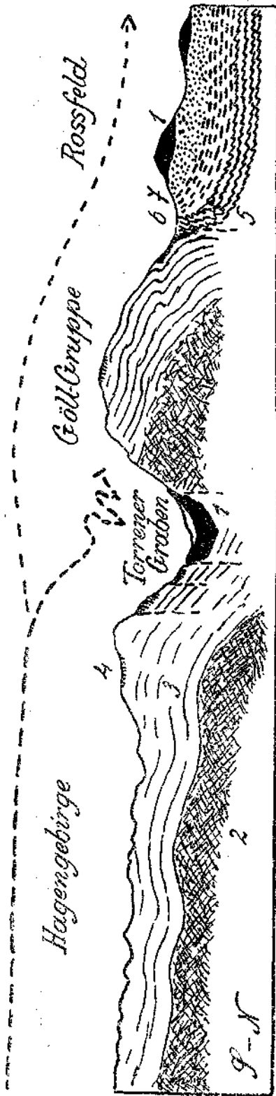
Fig. 13. 1 = Weifener Sch. + Haselgebirge + Ramsau D. + Muschelkalk + Hallstätter Sch. 2 = Ramsau D. + Raibler Sch. 3 = Dachsteinkalk — Dachsteindolomit — Dachsteinriffkalk. 4 = Lias. 5 = Oberalm Sch. 6 = Schrambach Sch. 7 = Roßfeld Sch.
