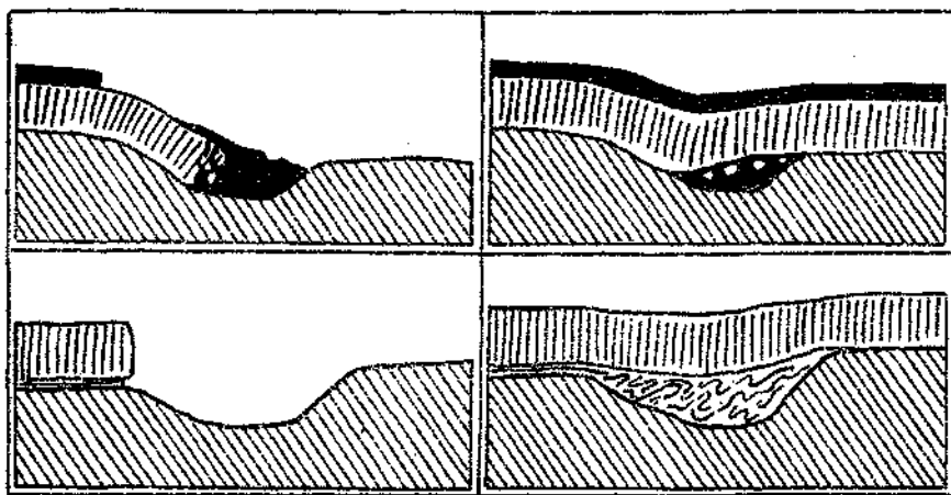
Fig. 9. Im oberen Fall Ausstopfung einer Kerbe durch abgerutschtes Hängendmaterial einer Schubmasse, im unteren Fall durch angeschopptes Liegendmaterial. Die Bewegung der Schubmassen erfolgt von links gegen rechts.
