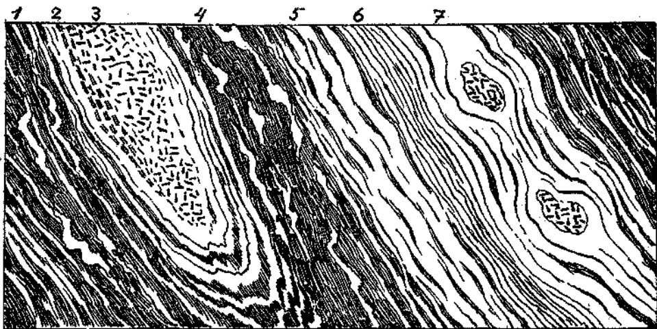
Fig. 8. Eklogit im Grieskar: 1 gebänderter Amphibolit mit Aplitadern, 2 streifig-lager Eklogit, 3 massiger hellbunter Eklogit, 4 dunkler Amphibolit mit Aplitadern, 5 grob weiß gefasertes Amphibolit, 6 feinflaseriger Amphibolit, 7 Eklogitknollen in Flaseramphibolit.
